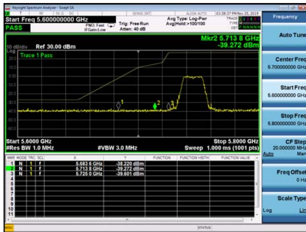
U-NII-3 Band Edge-802.11ac(20MHz) ,5745MHz
