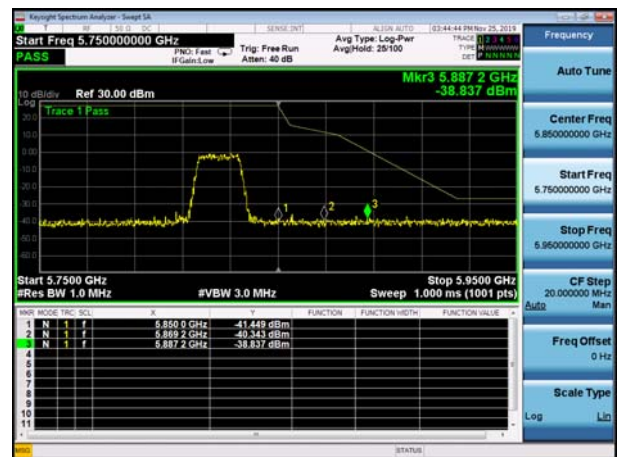
U-NII-3 Band Edge-802.11ac(40MHz) ,5795MHz
