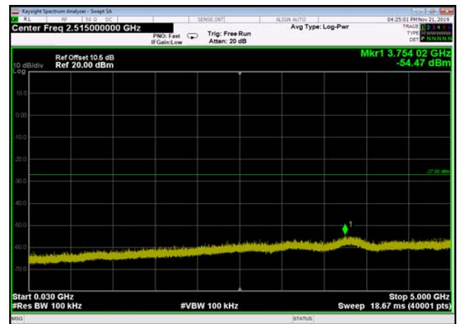
U-NII-2c ,Plot 2,30MHz~5000MHz-802.11 ac(40MHz),5510MHz,Ant1
