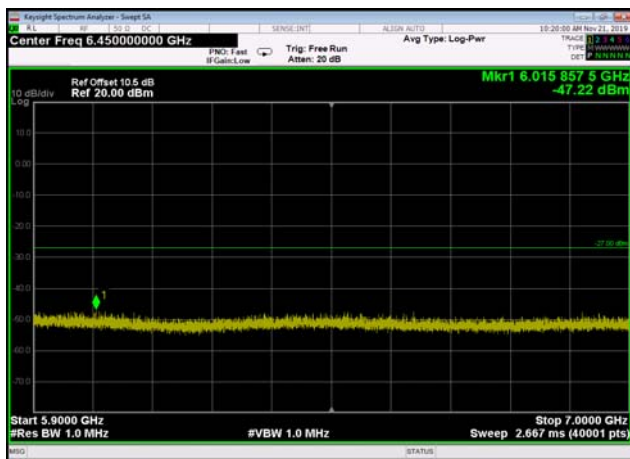
U-NII-2c ,Plot 3,5900MHz~7000MHz-802. 11a(20MHz),5700MHz,Ant1
