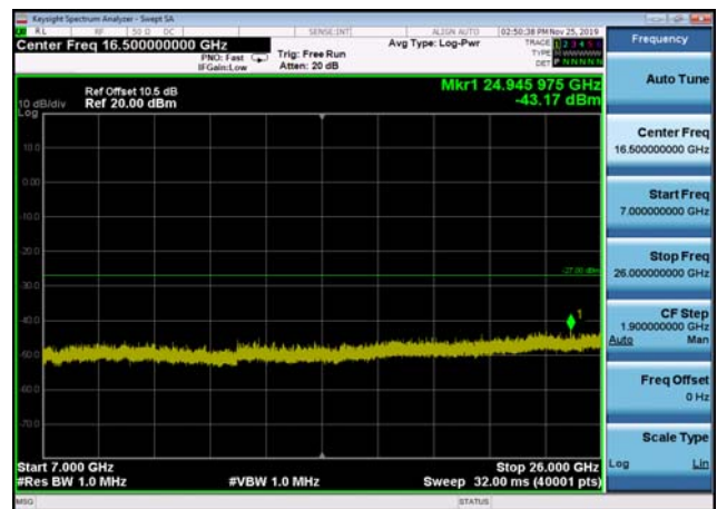
U-NII-3 ,Plot 4,7000MHz~26000MHz-802. 11ac(40MHz),5795MHz,Ant1
