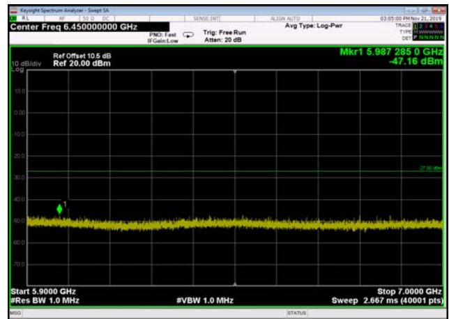
U-NII-2c ,Plot 3,5900MHz~7000MHz-802. 11ac(40MHz),5590MHz,Ant1
