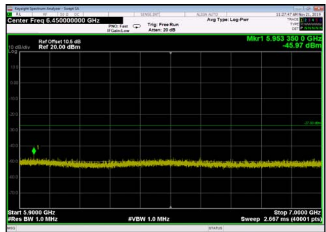
U-NII-2c ,Plot 3,5900MHz~7000MHz-802. 11ac(20MHz),5500MHz,Ant1
