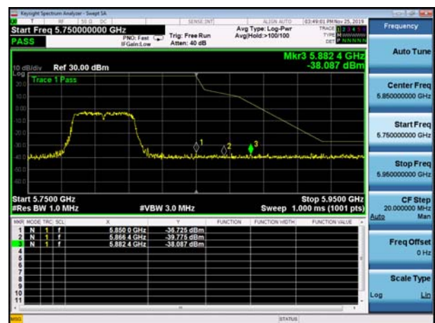
U-NII-3 Band Edge-802.11ac(40MHz) ,5795MHz
