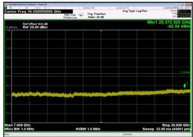
U-NII-2c ,Plot 4,7000MHz~26000MHz-802 .11ac(20MHz),5600MHz,Ant1
