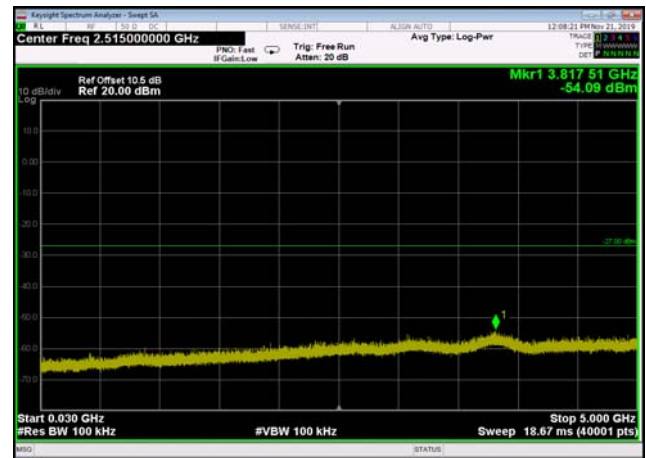
U-NII-2c ,Plot 2,30MHz~5000MHz-802.11 ac(20MHz),5600MHz,Ant1
