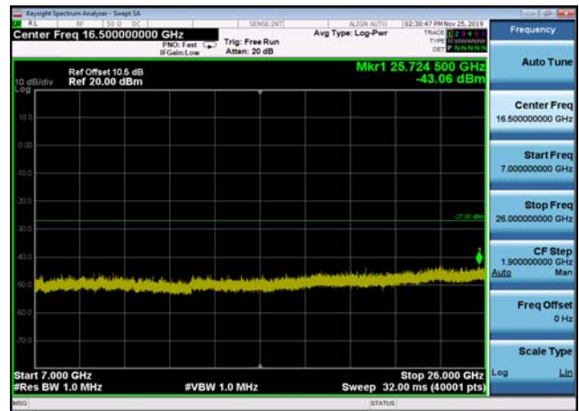
U-NII-3 ,Plot 4,7000MHz~26000MHz-802. 11ac(20MHz),5825MHz,Ant1
