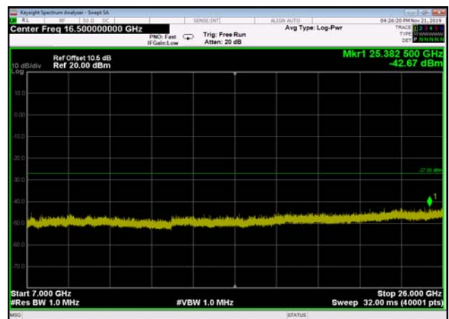
U-NII-2c ,Plot 4,7000MHz~26000MHz-802 .11ac(40MHz),5510MHz,Ant1
