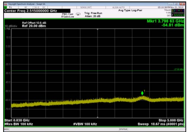
U-NII-3 ,Plot 2,30MHz~5000MHz-802.11a c(20MHz),5745MHz,Ant1
