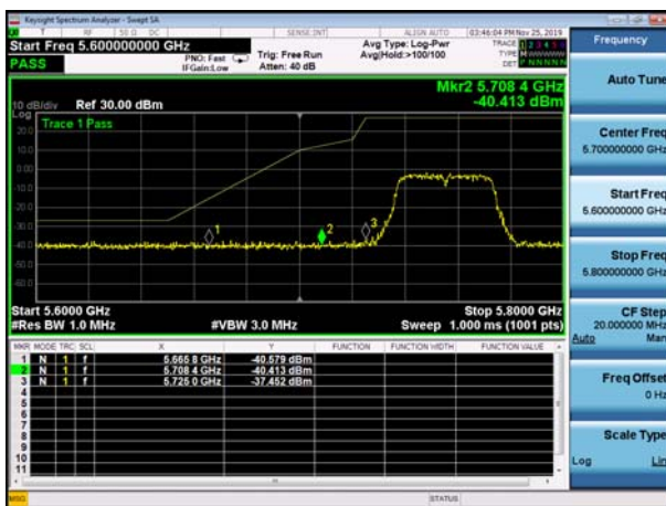
U-NII-3 Band Edge-802.11n(40MHz) ,5755MHz
