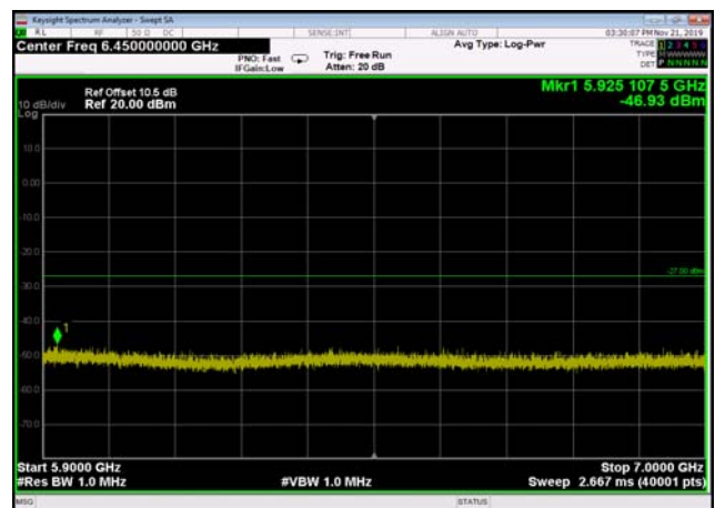
U-NII-2c ,Plot 3,5900MHz~7000MHz-802. 11ac(20MHz),5500MHz,Ant1
