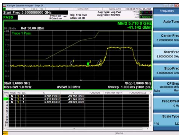
U-NII-3 Band Edge-802.11ac(40MHz) ,5755MHz
