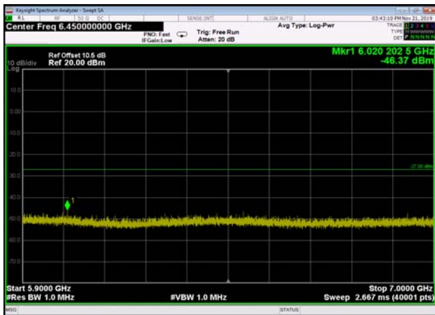
U-NII-2c ,Plot 3,5900MHz~7000MHz-802. 11n(40MHz),5670MHz,Ant1
