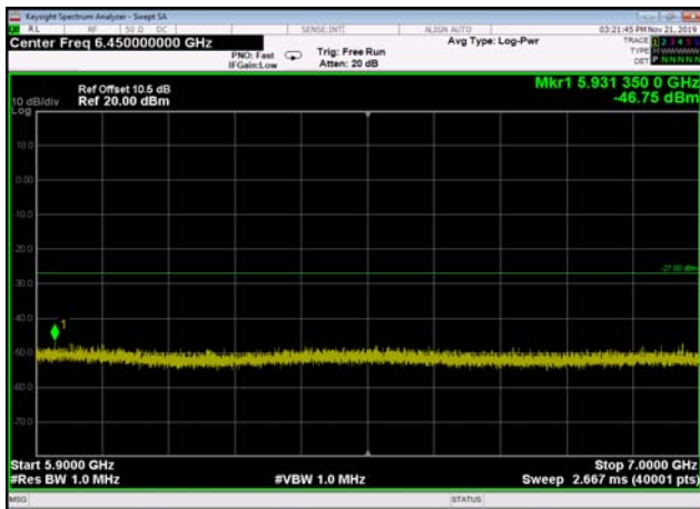
U-NII-2c ,Plot 3,5900MHz~7000MHz-802. 11ac(40MHz),5510MHz,Ant1
