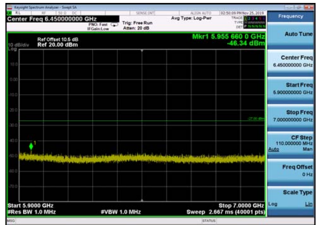
U-NII-3 ,Plot 3,5900MHz~7000MHz-802.1 1ac(40MHz),5795MHz,Ant1
