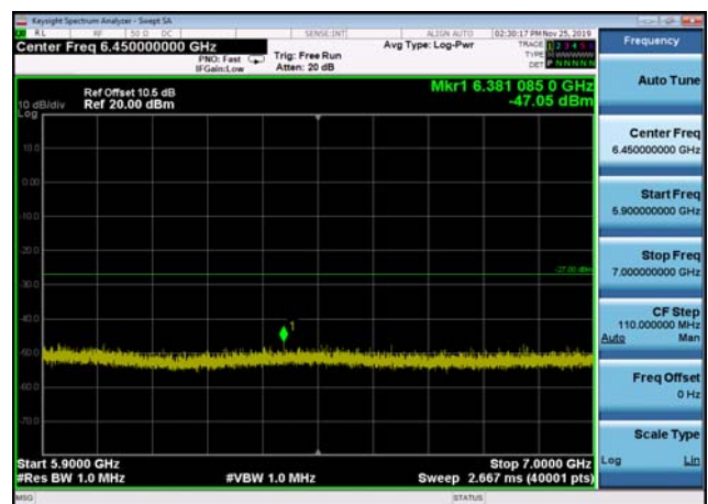
U-NII-3 ,Plot 3,5900MHz~7000MHz-802.1 1ac(20MHz),5745MHz,Ant1
