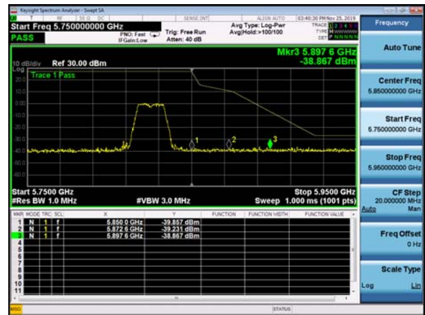
U-NII-3 Band Edge-802.11ac(20MHz) ,5825MHz
