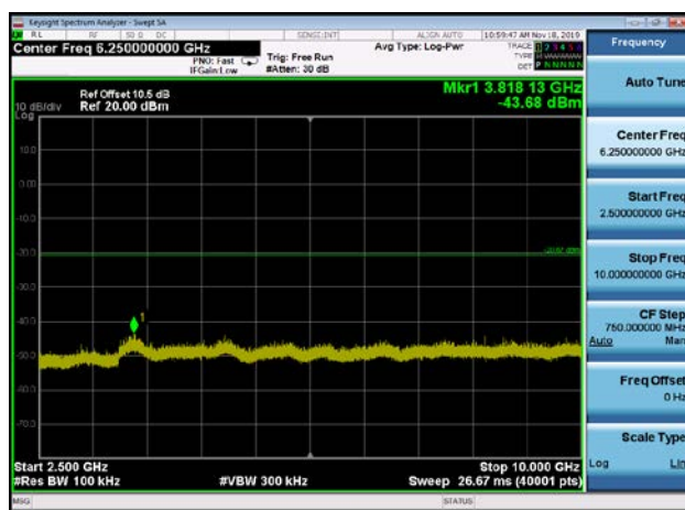
,Plot 4,2500MHz~10000MHz-802.11n(HT40 ) ,2452MHz,Ant0
