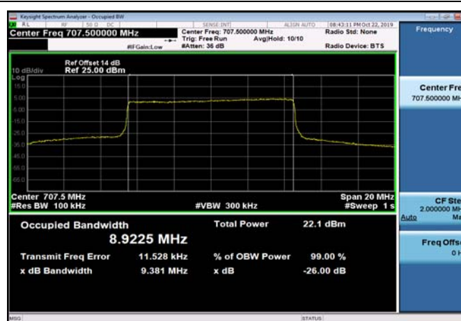
FDD12_MidRange_10MHz_707.5MHz_Q16
