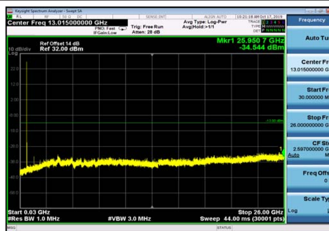
FDD17_HighRange_5MHz_30MHz~26GHz
