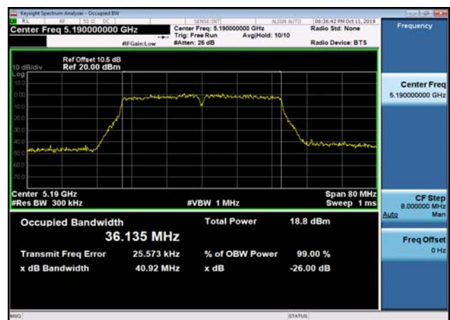
U-NII-1 26dB Bandwidth-802.11ac(40MHz) ,5190MHz,Ant2
