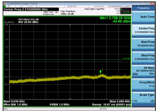
U-NII-1 ,Plot 2,30MHz~5000MHz-802.11n (20MHz),5220MHz,Ant2
