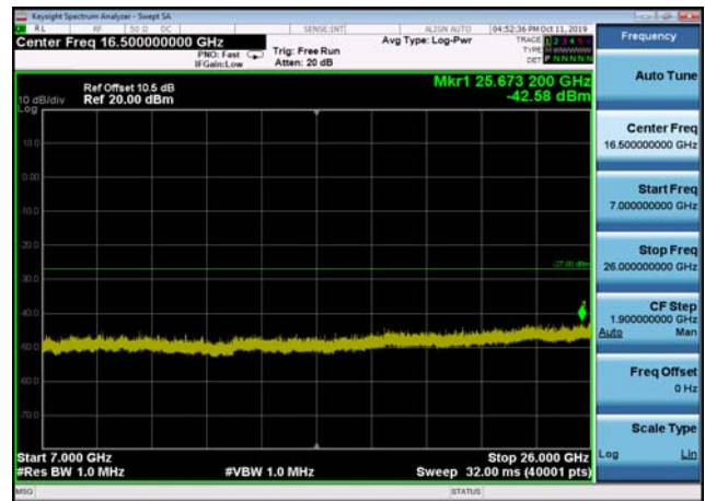
U-NII-1 ,Plot 4,7000MHz~26000MHz-802. 11n(40MHz),5230MHz,Ant2
