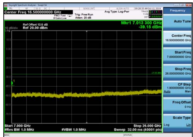
U-NII-2a ,Plot 4,7000MHz~26000MHz-802 .11n(20MHz),5300MHz,Ant2
