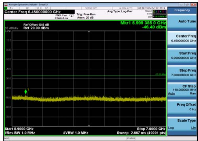
U-NII-2a ,Plot 3,5900MHz~7000MHz-802. 11ac(40MHz),5270MHz,Ant2
