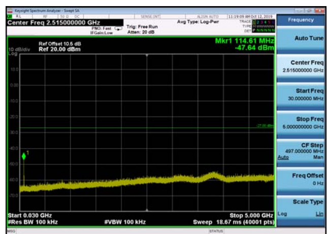
U-NII-2a ,Plot 2,30MHz~5000MHz-802.11 ac(40MHz),5270MHz,Ant2
