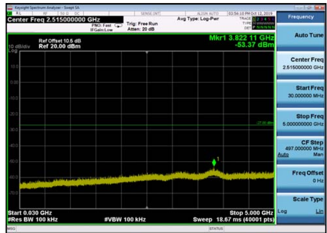
U-NII-2a ,Plot 2,30MHz~5000MHz-802.11 n(40MHz),5310MHz,Ant2
