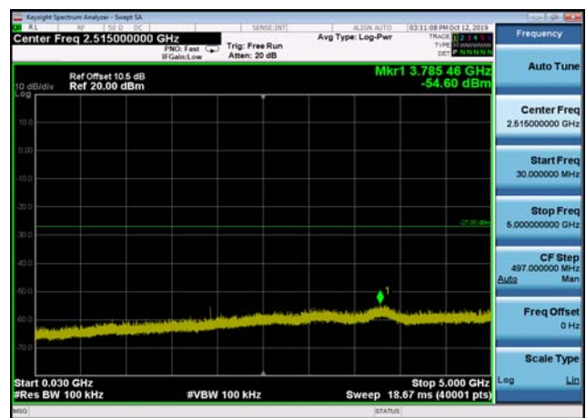
U-NII-2a ,Plot 2,30MHz~5000MHz-802.11 ac(20MHz),5260MHz,Ant2
