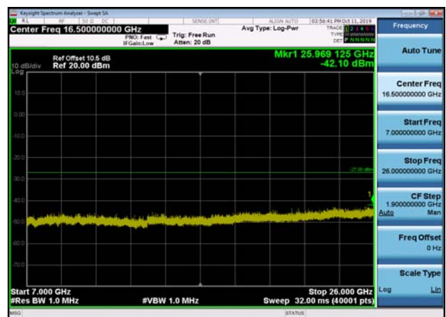
U-NII-1 ,Plot 4,7000MHz~26000MHz-802. 11ac(20MHz),5180MHz,Ant2
