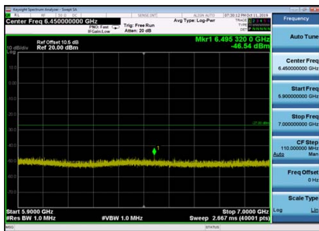
U-NII-2a ,Plot 3,5900MHz~7000MHz-802. 11a(20MHz),5300MHz,Ant2
