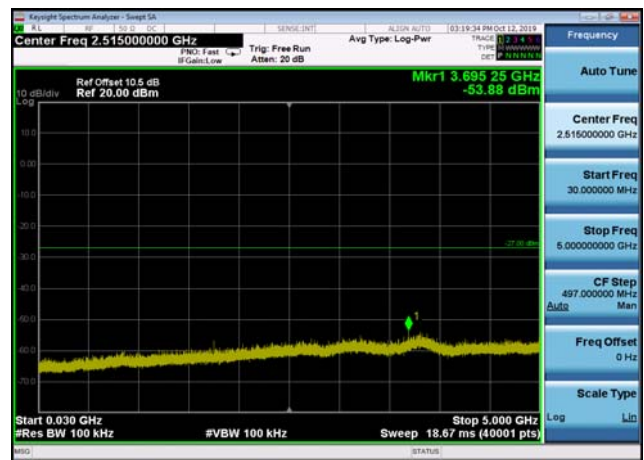
U-NII-2a ,Plot 2,30MHz~5000MHz-802.11 ac(20MHz),5320MHz,Ant2
