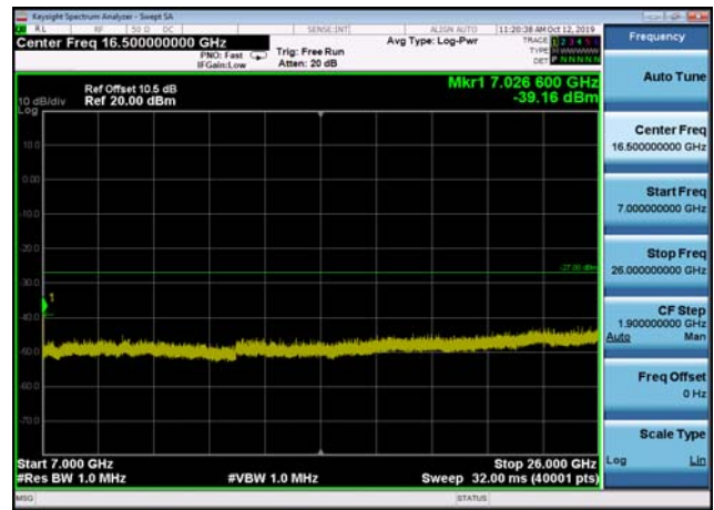
U-NII-2a ,Plot 4,7000MHz~26000MHz-802 .11ac(40MHz),5310MHz,Ant2
