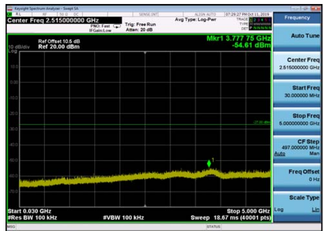
U-NII-2a ,Plot 2,30MHz~5000MHz-802.11 a(20MHz),5320MHz,Ant2
