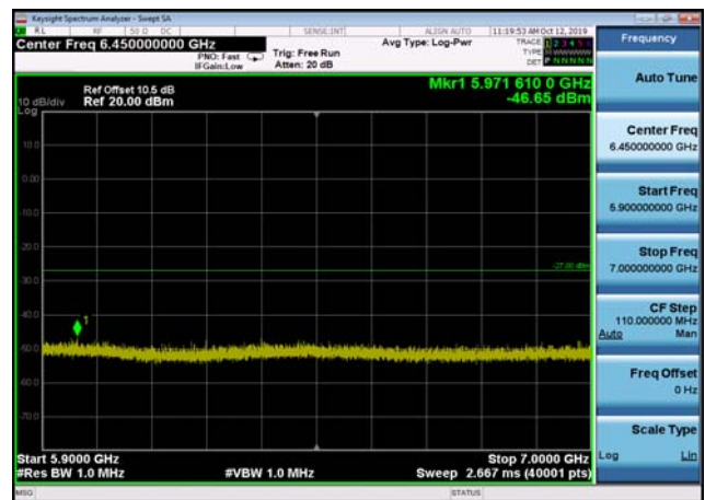
U-NII-2a ,Plot 3,5900MHz~7000MHz-802. 11ac(40MHz),5310MHz,Ant2
