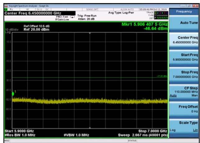
U-NII-2c ,Plot 3,5900MHz~7000MHz-802.11 n(20MHz),5500MHz,Ant2
