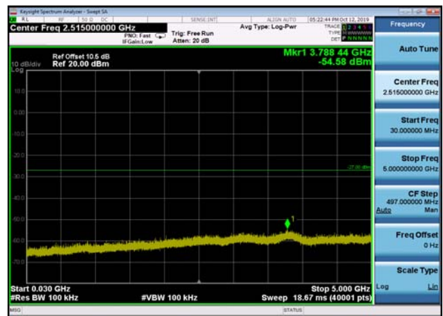
U-NII-2c ,Plot 2,30MHz~5000MHz-802.11 n(20MHz),5700MHz,Ant2
