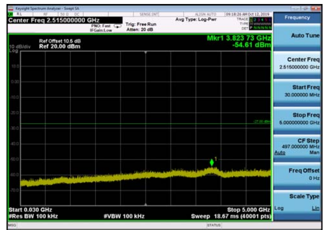
U-NII-2a ,Plot 2,30MHz~5000MHz-802.11 n(20MHz),5300MHz,Ant2
