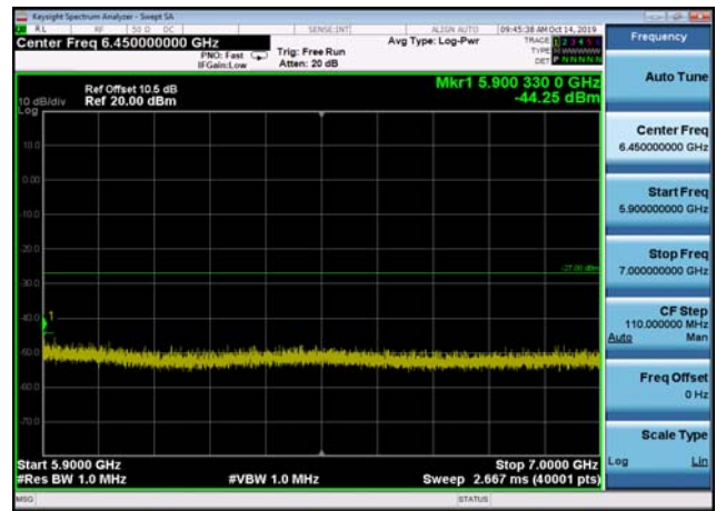
U-NII-3 ,Plot 3,5900MHz~7000MHz-802.1 1n(20MHz),5825MHz,Ant2
