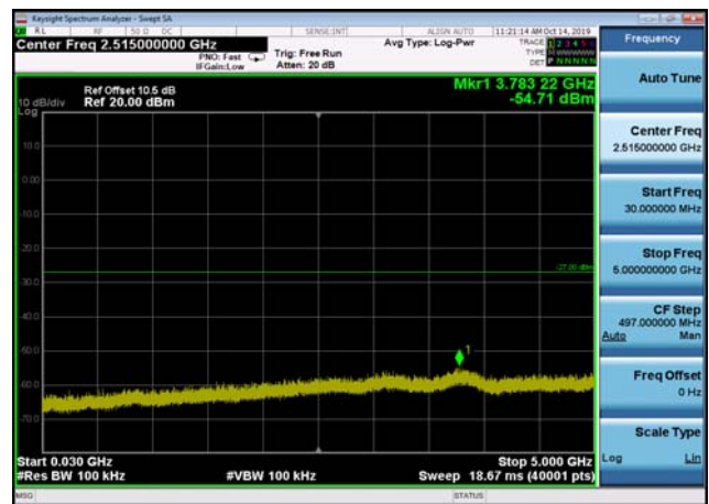
U-NII-3 ,Plot 2,30MHz~5000MHz-802.11n (40MHz),5795MHz,Ant2
