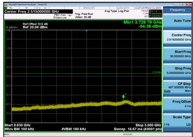
U-NII-2c ,Plot 2,30MHz~5000MHz-802.11 ac(40MHz),5670MHz,Ant2
