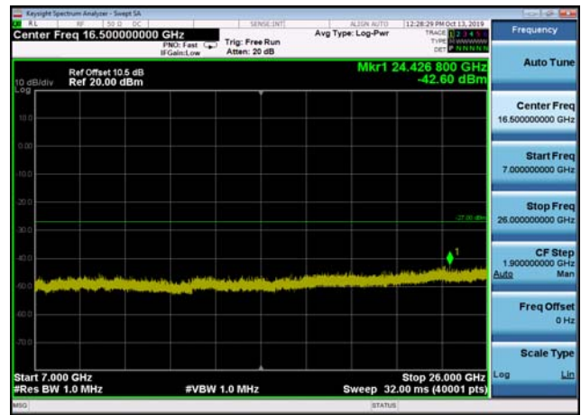
U-NII-2c ,Plot 4,7000MHz~26000MHz-802 .11ac(40MHz),5670MHz,Ant2
