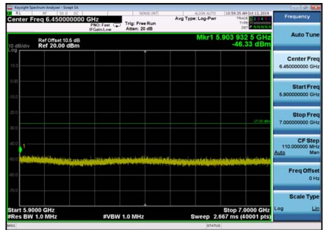
U-NII-2c ,Plot 3,5900MHz~7000MHz-802. 11n(40MHz),5670MHz,Ant2
