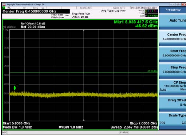
U-NII-2c ,Plot 3,5900MHz~7000MHz-802. 11ac(20MHz),5700MHz,Ant1
