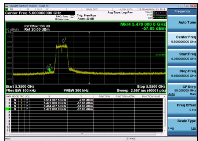
U-NII-2c ,Plot 1,Band Edge-802.11ac(4 0MHz),5510MHz,Ant2
