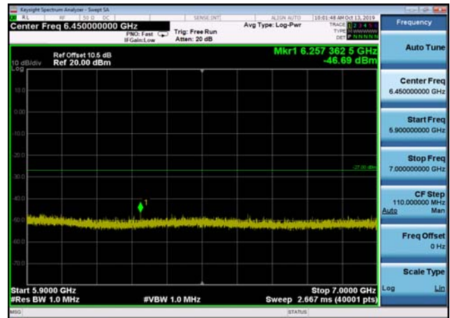
U-NII-2c ,Plot 3,5900MHz~7000MHz-802. 11ac(40MHz),5510MHz,Ant2
