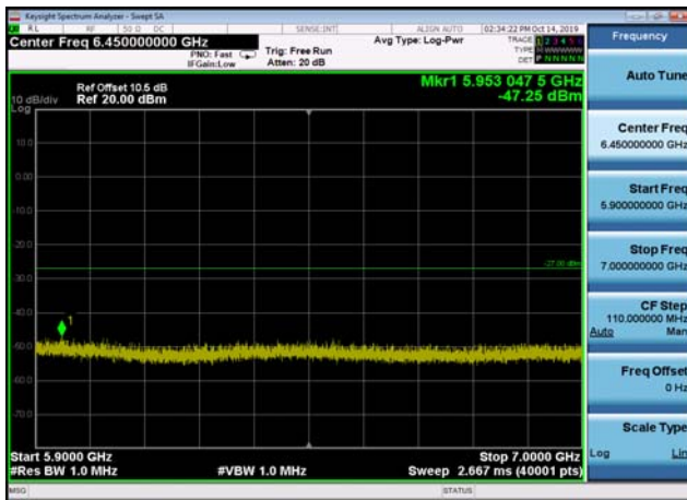
U-NII-3 ,Plot 3,5900MHz~7000MHz-802.1 1n(40MHz),5795MHz,Ant1
