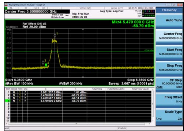
U-NII-2c ,Plot 1,Band Edge-802.11ac(20 MHz),5500MHz,Ant2
