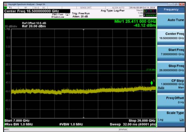
U-NII-3 ,Plot 4,7000MHz~26000MHz-802. 11n(20MHz),5825MHz,Ant2
