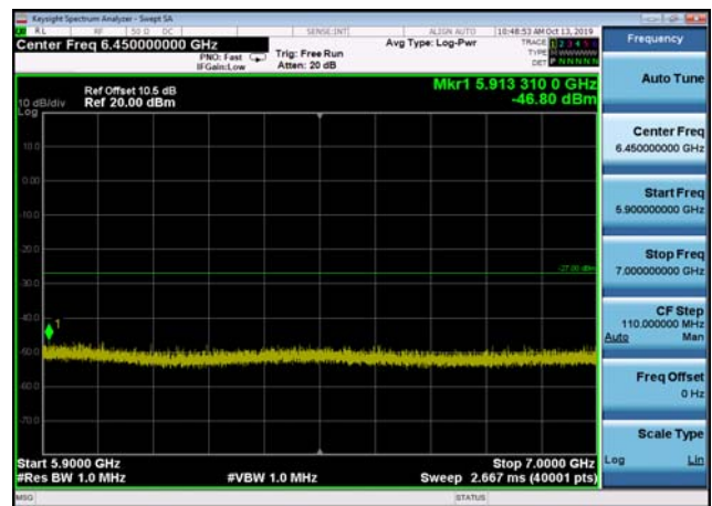
U-NII-2c ,Plot 3,5900MHz~7000MHz-802. 11n(40MHz),5510MHz,Ant2
