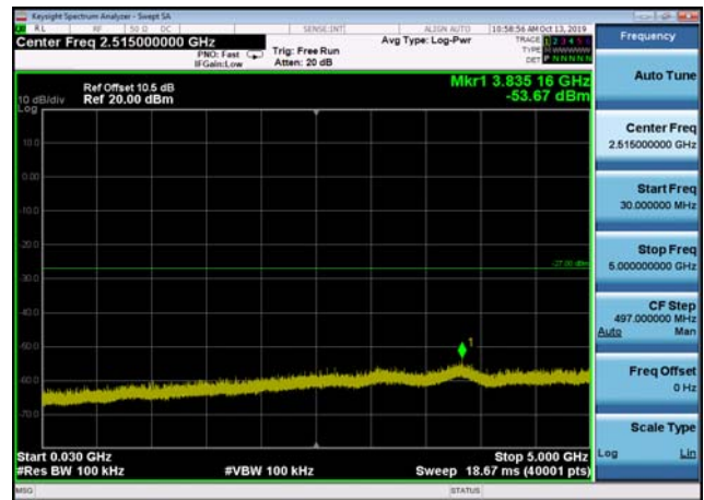
U-NII-2c ,Plot 2,30MHz~5000MHz-802.11 n(40MHz),5670MHz,Ant2
