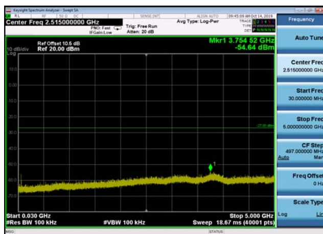
U-NII-3 ,Plot 2,30MHz~5000MHz-802.11n (20MHz),5825MHz,Ant2
