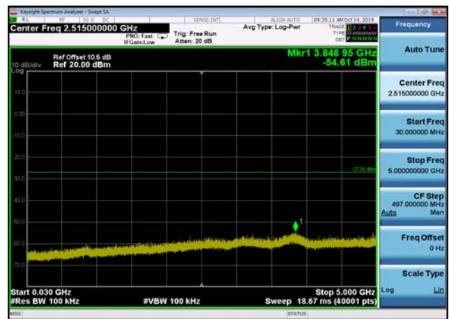
U-NII-3 ,Plot 2,30MHz~5000MHz-802.11n (20MHz),5745MHz,Ant2
