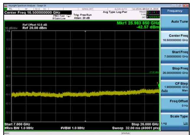
U-NII-3 ,Plot 4,7000MHz~26000MHz-802. 11n(40MHz),5755MHz,Ant2
