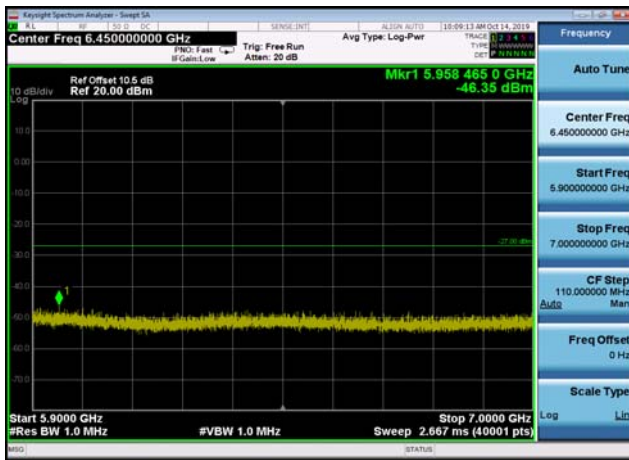
U-NII-3 ,Plot 3,5900MHz~7000MHz-802.1 1n(20MHz),5825MHz,Ant1
