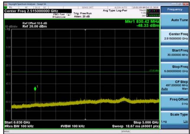
U-NII-2c ,Plot 2,30MHz~5000MHz-802.11 ac(40MHz),5510MHz,Ant2
