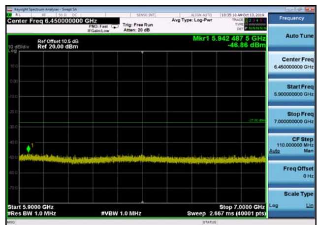
U-NII-2c ,Plot 3,5900MHz~7000MHz-802. 11ac(20MHz),5500MHz,Ant2
