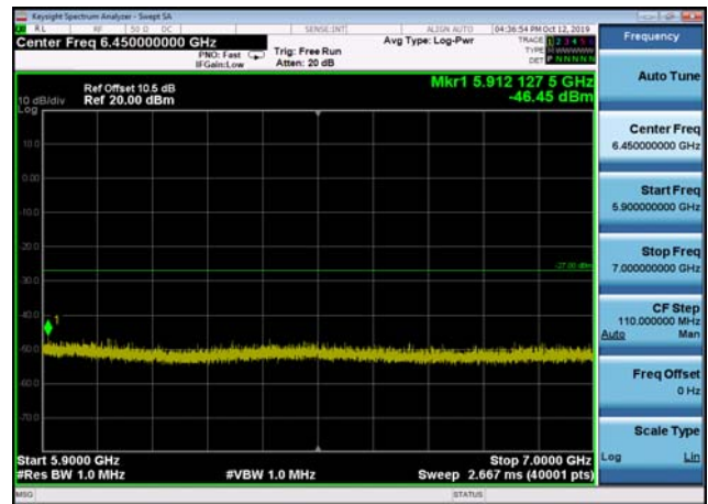
U-NII-2c ,Plot 3,5900MHz~7000MHz-802. 11a(20MHz),5700MHz,Ant2
