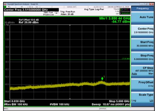
U-NII-2c ,Plot 2,30MHz~5000MHz-802.11 a(20MHz),5500MHz,Ant2
