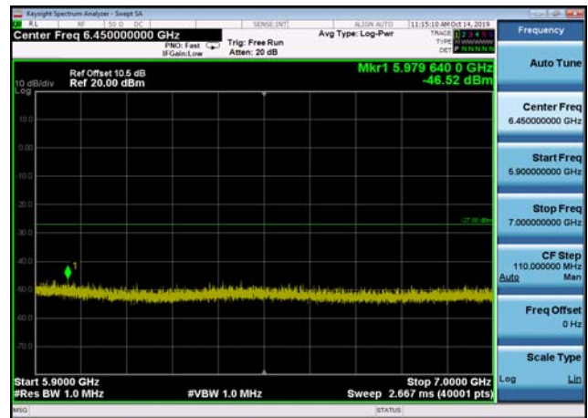
U-NII-3 ,Plot 3,5900MHz~7000MHz-802.1 1n(40MHz),5795MHz,Ant2
