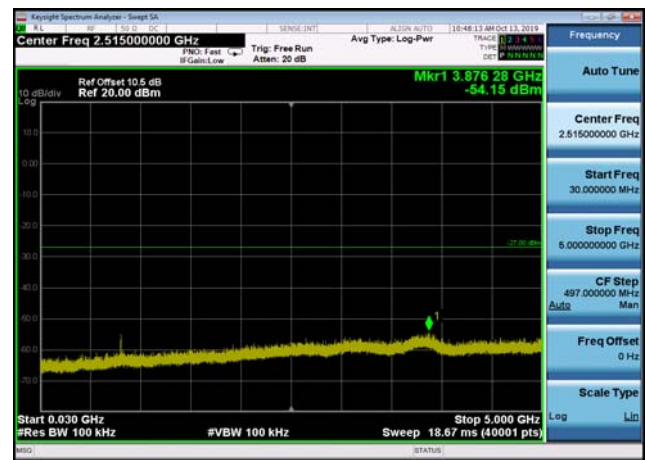
U-NII-2c ,Plot 2,30MHz~5000MHz-802.11 n(40MHz),5510MHz,Ant2
