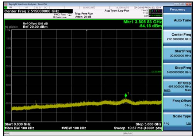
U-NII-2c ,Plot 2,30MHz~5000MHz-802.11 ac(20MHz),5500MHz,Ant2
