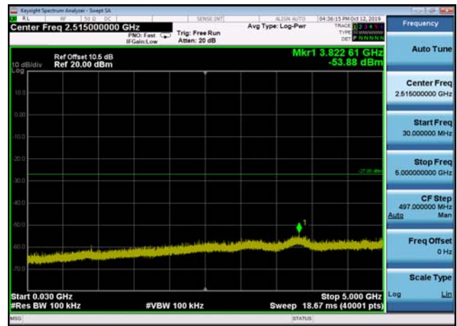
U-NII-2c ,Plot 2,30MHz~5000MHz-802.11 a(20MHz),5700MHz,Ant2
