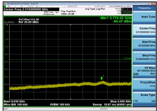
U-NII-2c ,Plot 2,30MHz~5000MHz-802.11 ac(20MHz),5700MHz,Ant2
