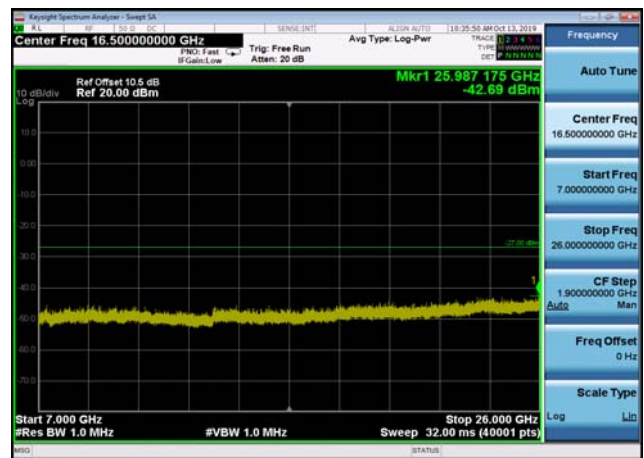
U-NII-2c ,Plot 4,7000MHz~26000MHz-802 .11ac(20MHz),5500MHz,Ant2
