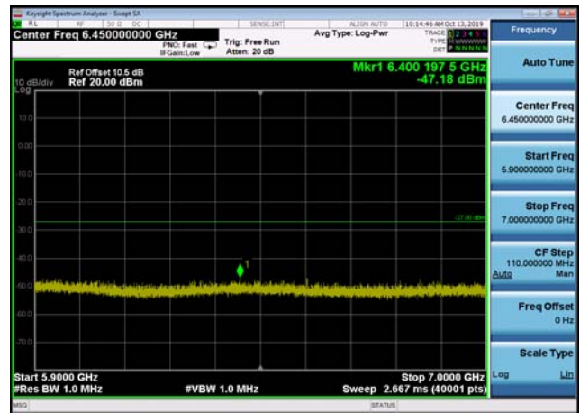
U-NII-2c ,Plot 3,5900MHz~7000MHz-802. 11ac(20MHz),5700MHz,Ant2
