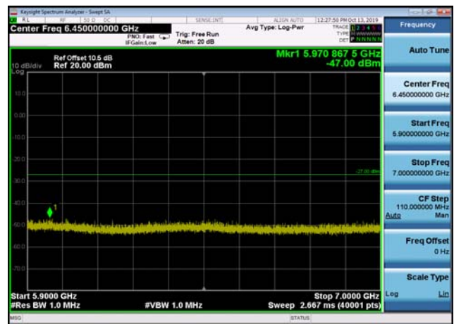
U-NII-2c ,Plot 3,5900MHz~7000MHz-802. 11ac(40MHz),5670MHz,Ant2
