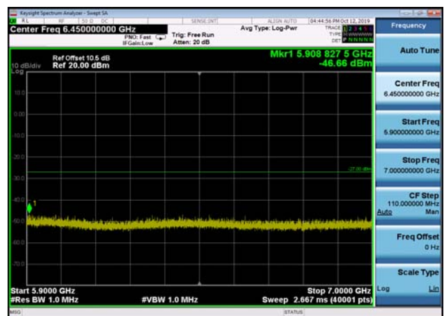
U-NII-2c ,Plot 3,5900MHz~7000MHz-802. 11a(20MHz),5500MHz,Ant2
