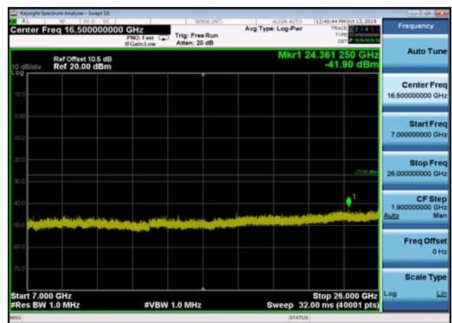
U-NII-2c ,Plot 4,7000MHz~26000MHz-802 .11ac(40MHz),5510MHz,Ant2
