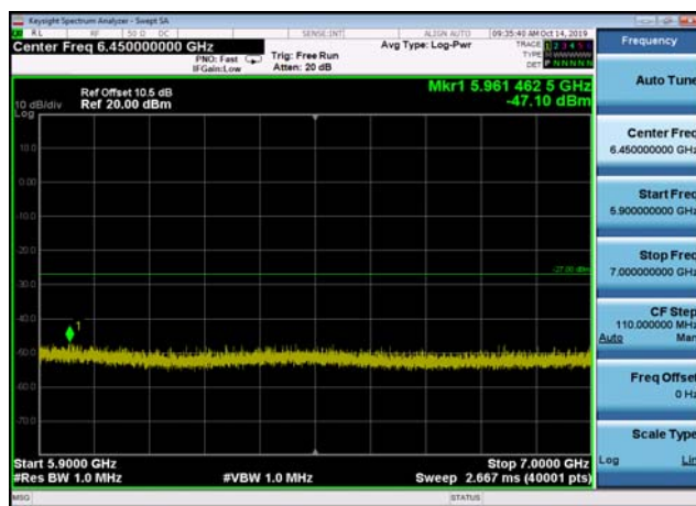
U-NII-3 ,Plot 3,5900MHz~7000MHz-802.1 1n(20MHz),5745MHz,Ant2
