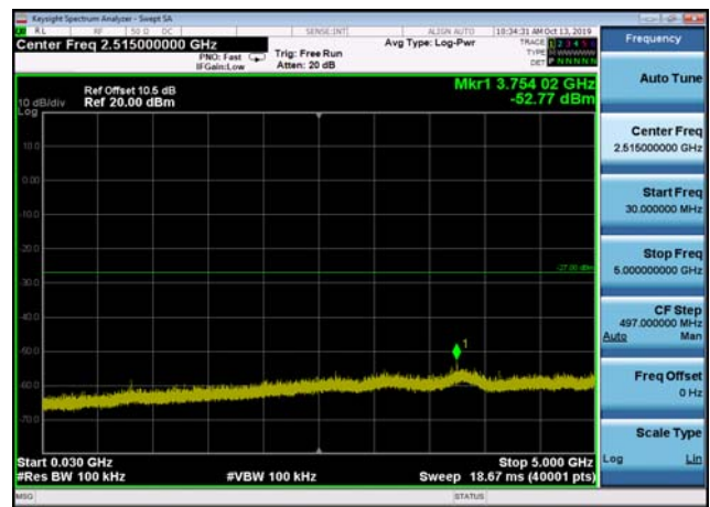
U-NII-2c ,Plot 2,30MHz~5000MHz-802.11 ac(20MHz),5500MHz,Ant2
