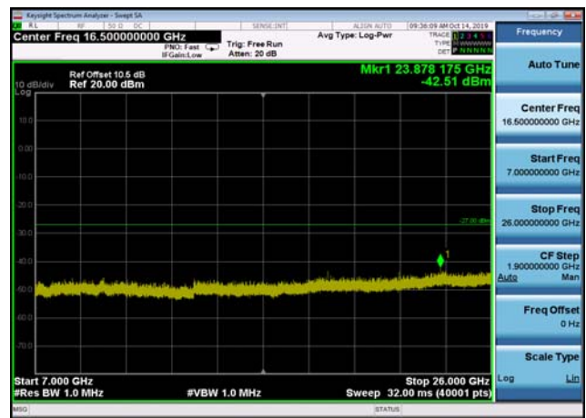
U-NII-3 ,Plot 4,7000MHz~26000MHz-802. 11n(20MHz),5745MHz,Ant2
