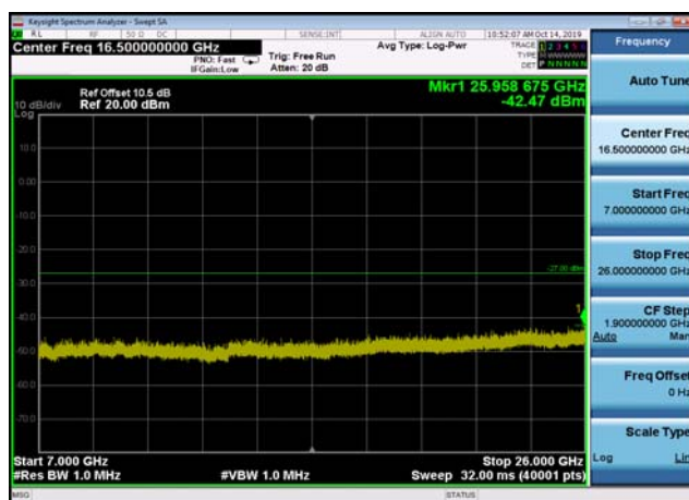
U-NII-3 ,Plot 4,7000MHz~26000MHz-802. 11ac(40MHz),5755MHz,Ant2
