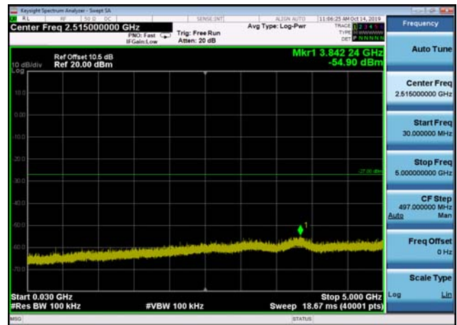
U-NII-3 ,Plot 2,30MHz~5000MHz-802.11a c(20MHz),5785MHz,Ant2
