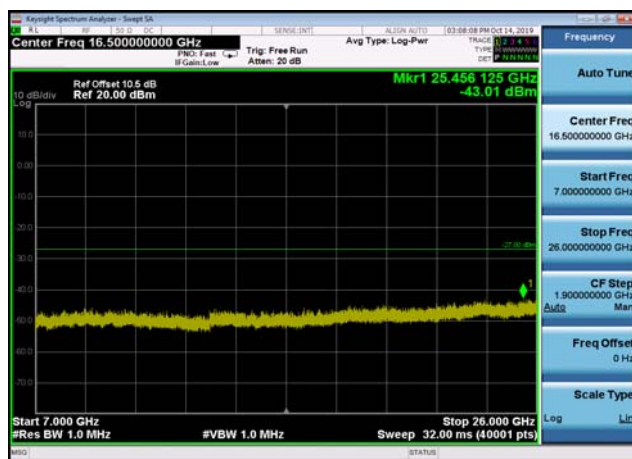
U-NII-3 ,Plot 4,7000MHz~26000MHz-802. 11ac(40MHz),5795MHz,Ant2
