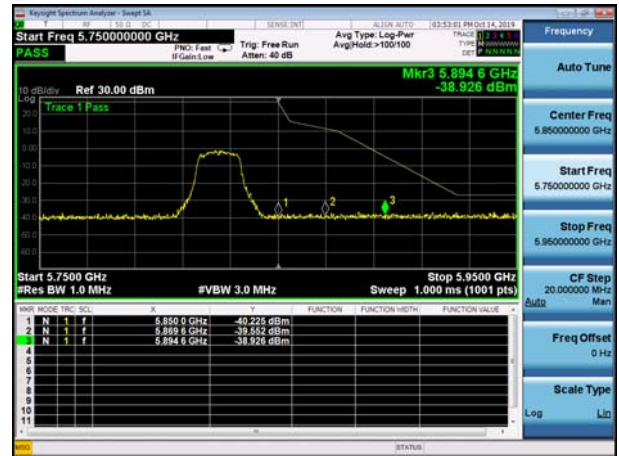
U-NII-3 ,Plot 1,Band Edge-802.11ac(40 MHz),5755MHz,Ant2
