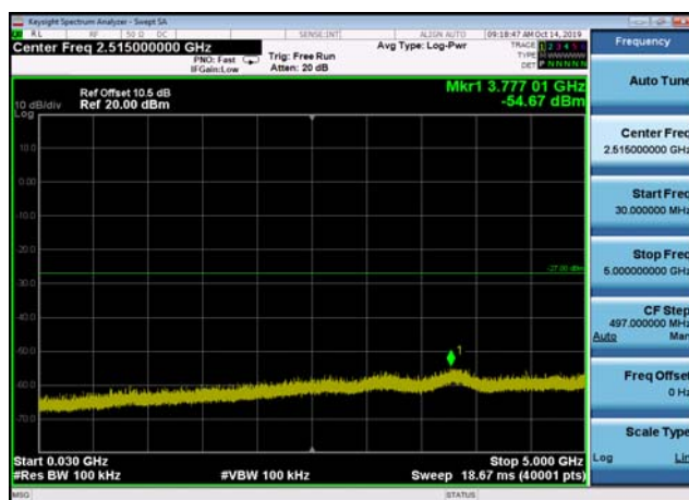
U-NII-3 ,Plot 2,30MHz~5000MHz-802.11a (20MHz),5785MHz,Ant2
