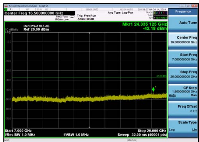
U-NII-3 ,Plot 4,7000MHz~26000MHz-802. 11ac(20MHz),5785MHz,Ant2
