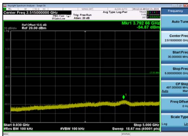
U-NII-3 ,Plot 2,30MHz~5000MHz-802.11a (20MHz),5825MHz,Ant2
