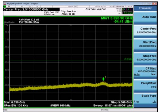
U-NII-3 ,Plot 2,30MHz~5000MHz-802.11a c(40MHz),5795MHz,Ant2
