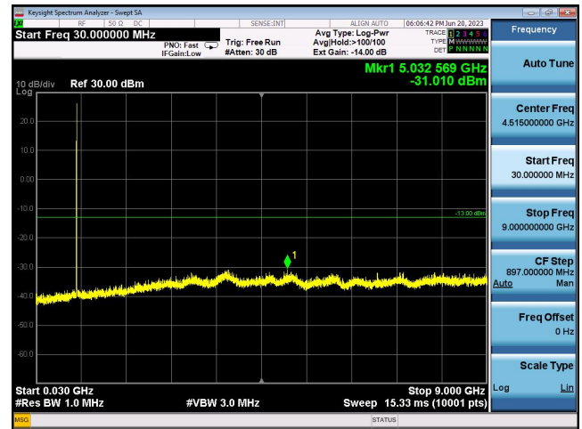
CDMA2000 BC0-384, 30MHz ~9GHz
