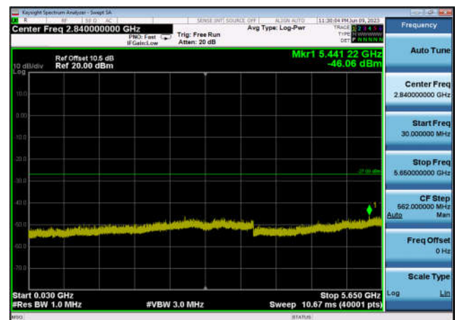
U-NII-3 ,Plot 2,30MHz~5650MHz-802.11a (20MHz),5785MHz,Ant1
