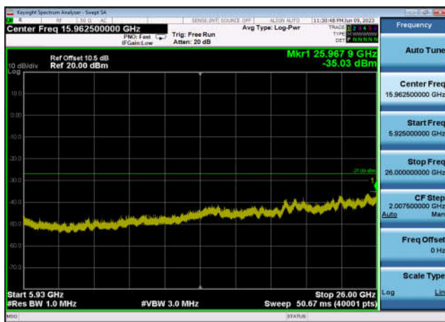
U-NII-3 ,Plot 3,5925MHz~26000MHz-802.11ac(20MHz),5745MHz,Ant1
