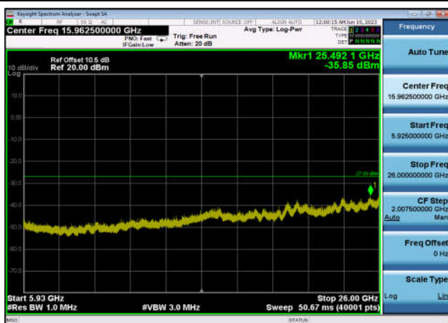
U-NII-3 ,Plot 3,5925MHz~26000MHz-802. 11n(20MHz),5745MHz,Ant1
