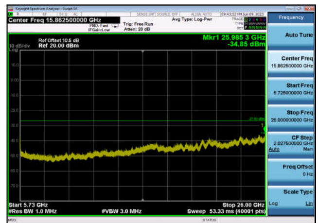
U-NII-2c ,Plot 3,5725MHz~26000MHz-802 .11ac(40MHz),5590MHz,Ant1
