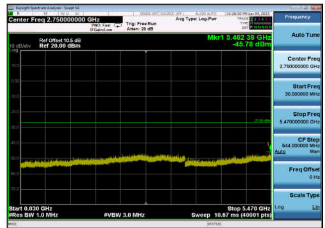
U-NII-2c ,Plot 2,30MHz~5470MHz-802.11 ac(80MHz),5610MHz,Ant1
