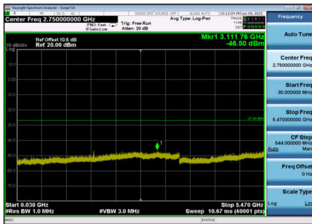
U-NII-2c ,Plot 2,30MHz~5470MHz-802.11 ac(80MHz),5530MHz,Ant1
