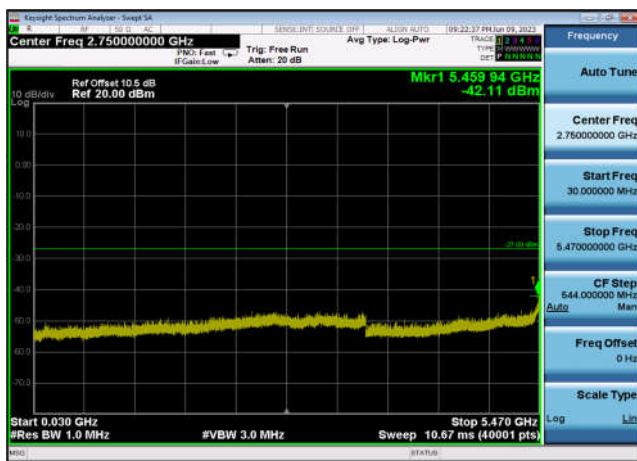
U-NII-2c ,Plot 2,30MHz~5470MHz-802.11 ac(20MHz),5700MHz,Ant1
