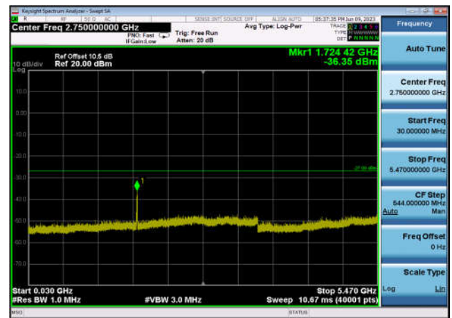
U-NII-2c ,Plot 2,30MHz~5470MHz-802.11 ac(20MHz),5600MHz,Ant1
