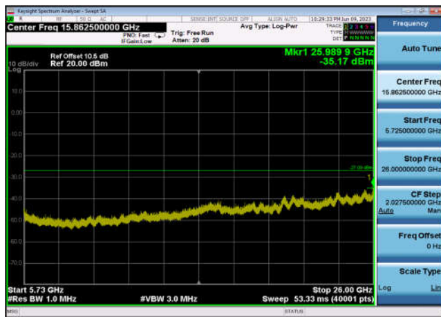
U-NII-2c ,Plot 3,5725MHz~26000MHz-802 .11ac(80MHz),5610MHz,Ant1
