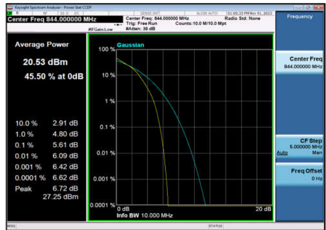
FDD05_HighRange_10MHz_844_fullRB _Q16
