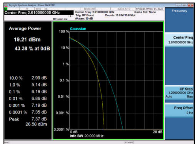
TDD38_HighRange_20MHz_2610_fullIRB _Q16
