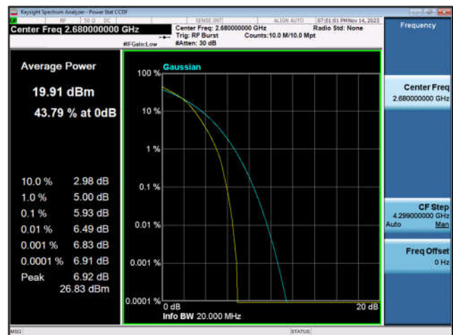
TDD41_HighRange_20MHz_2680_fullIRB _Q16
