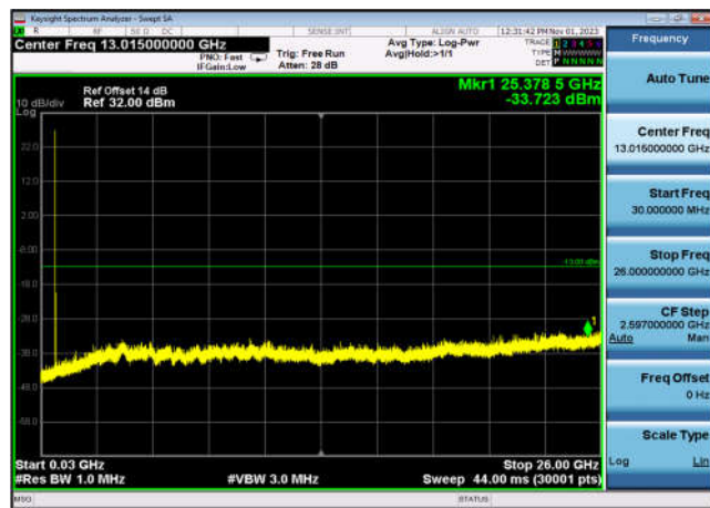
FDD17_HighRange_10MHz_30MHz~26GHz
