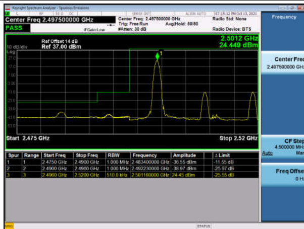
TDD7_20M Low FullIRB QPSK
