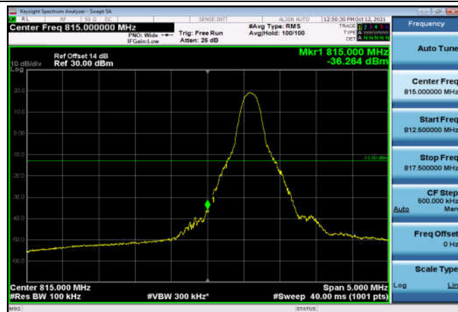
LowRange_ FDD26_10MHz_820_fullRB Low Q16
