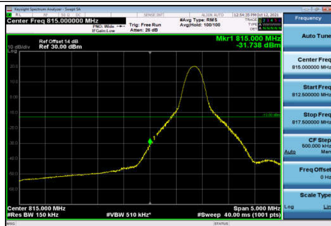
LowRange_FDD26_15MHz_822.5_OneRB low Q16
