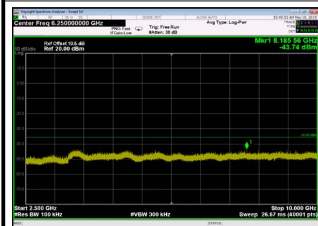
802.11n(HT40),2452MHz,Ant0,Plot 4,2500MHz~10000MHz
