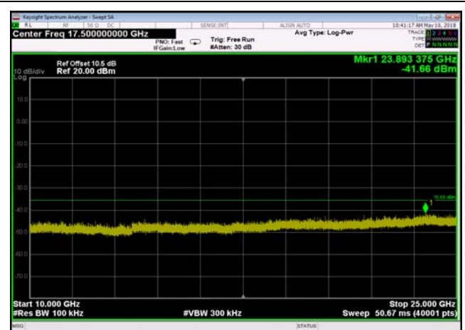
802.11n(HT40),2452MHz,Ant0,Plot 5,10000MHz~25000MHz
