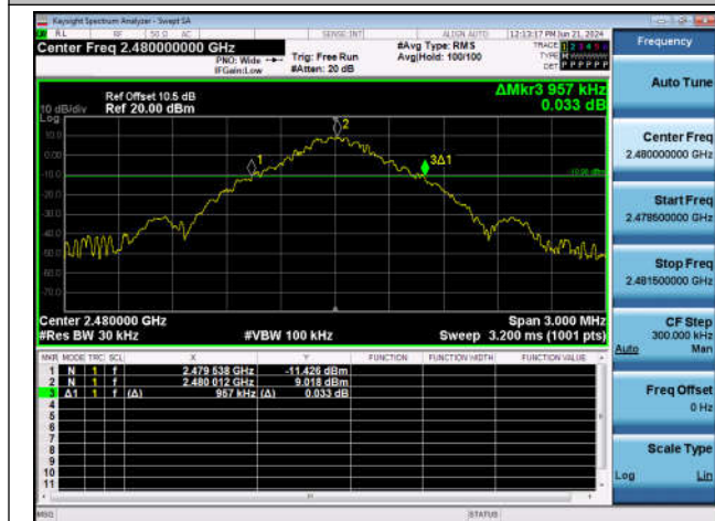
DH5-Ant1-2480
