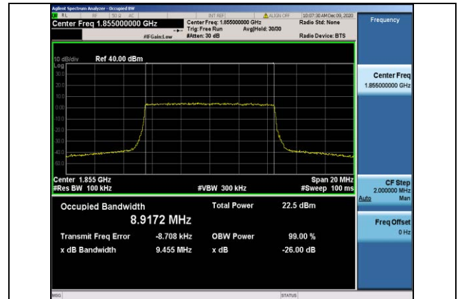
Band2-10MHz-QPSK-18650-50RB#0-8.9172
