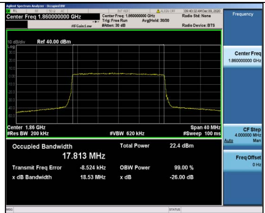
Band2-20MHz-QPSK-18700-100RB#0-17.813
