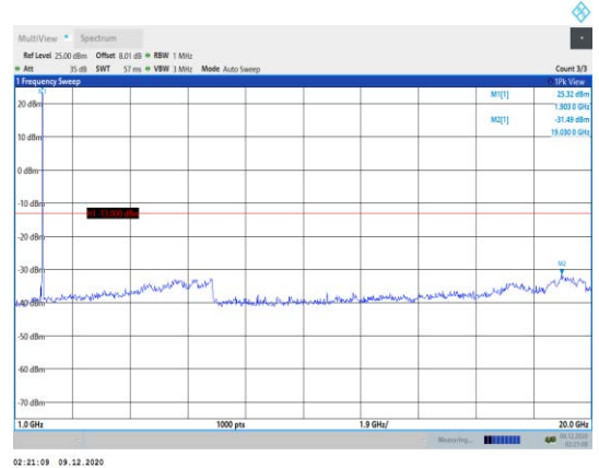
Band2-10MHz-QPSK-19150-1RB#0- Range2:1000~20000MHz
