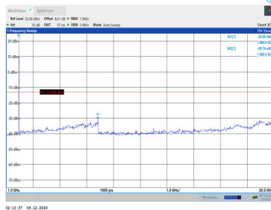
Band2-3MHz-QPSK-18900-1RB#0- Range2:1000~20000MHz
