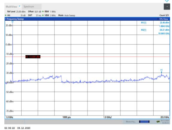
Band2-1.4MHz-QPSK-18900-1RB#0- Range2:1000~20000MHz
