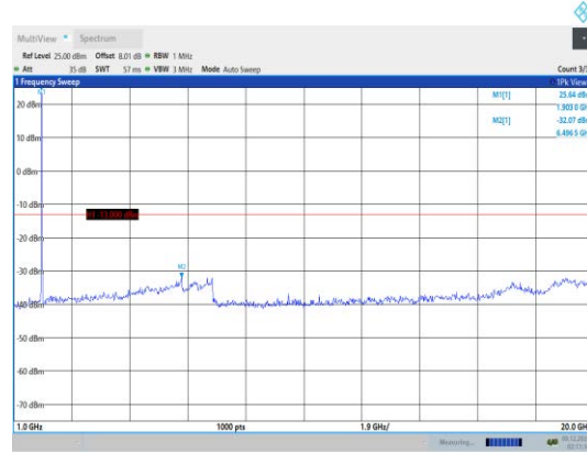
Band2-3MHz-QPSK-19185-1RB#0- Range2:1000~20000MHz
