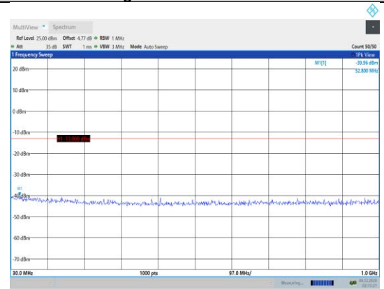
Band2-5MHz-QPSK-19175-1RB#0- Range1:30~1000MHz
