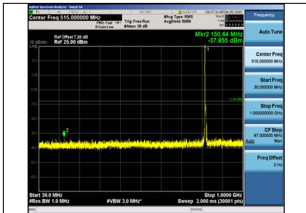
Band26-5MHz-QPSK-26765-1RB#0- Range1:30~1000MHz
