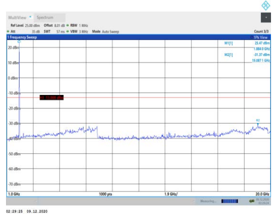
Band2-20MHz-QPSK-19100-1RB#0- Range2:1000~20000MHz
