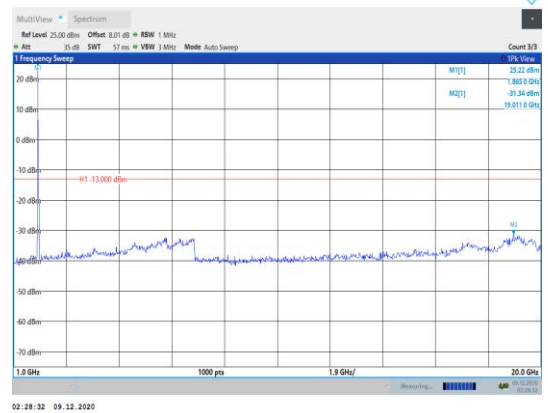
Band2-20MHz-QPSK-18900-1RB#0- Range2:1000~20000MHz
