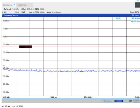
Band2-20MHz-QPSK-18700-1RB#0- Range1:30~1000MHz
