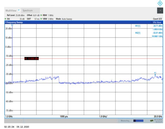
Band2-15MHz-QPSK-19125-1RB#0- Range2:1000~20000MHz
