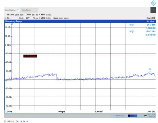
Band2-1.4MHz-QPSK-19193-1RB#0- Range2:1000~20000MHz
