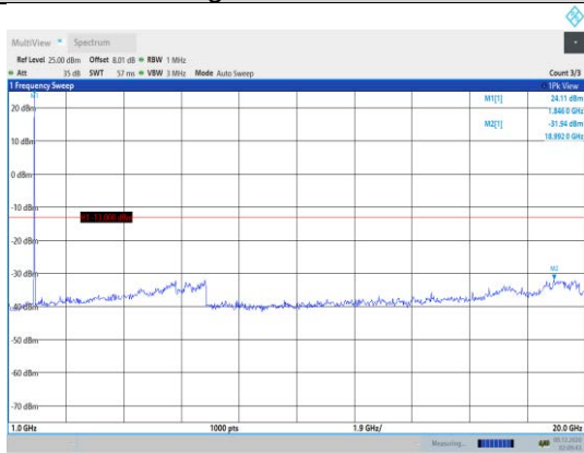
Band2-3MHz-QPSK-18615-1RB#0- Range2:1000~20000MHz
