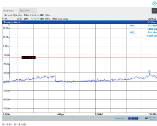
Band2-20MHz-QPSK-18700-1RB#0- Range2:1000~20000MHz
