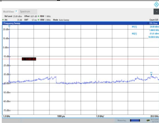
Band2-5MHz-QPSK-18625-1RB#0- Range2:1000~20000MHz
