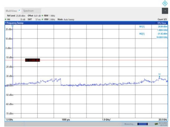
Band2-5MHz-QPSK-19175-1RB#0- Range2:1000~20000MHz
