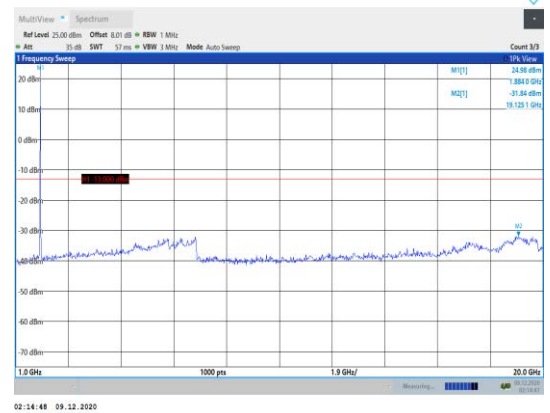
Band2-5MHz-QPSK-18900-1RB#0- Range2:1000~20000MHz
