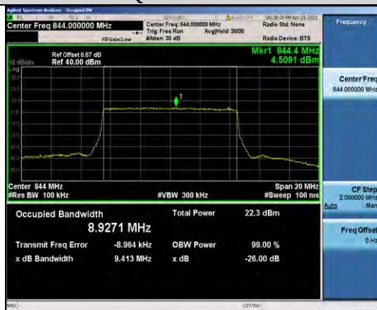
Band5-10MHz-QPSK-20600-50RB#0-8.9271
