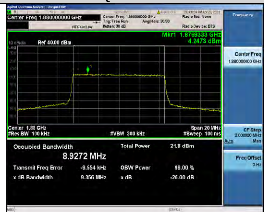
Band2-10MHz-16QAM-18900-50RB#0-8.9272
