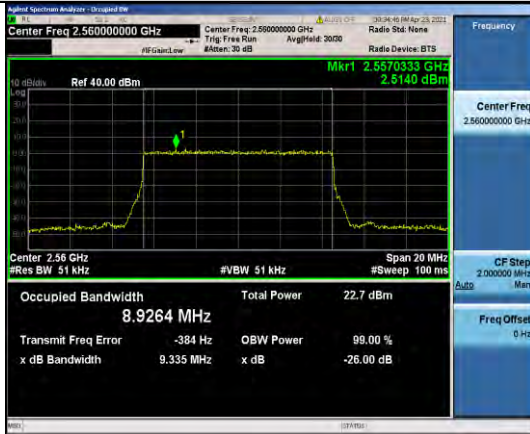
Band41-10MHz-QPSK-40290-50RB#0-8.9264
