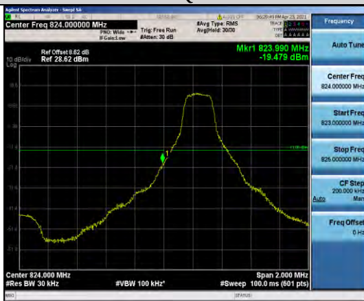
Band5-3MHz-QPSK-20415-1RB#0
