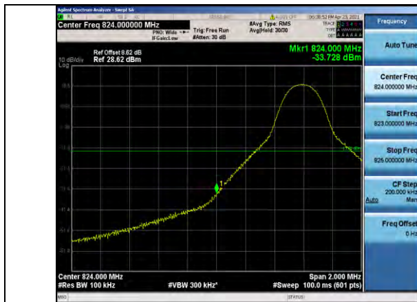
Band5-10MHz-QPSK-20450-1RB#0
