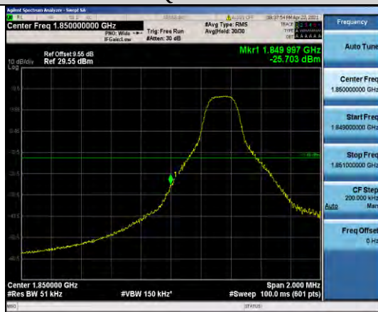
Band2-5MHz-16QAM-18625-1RB#0
