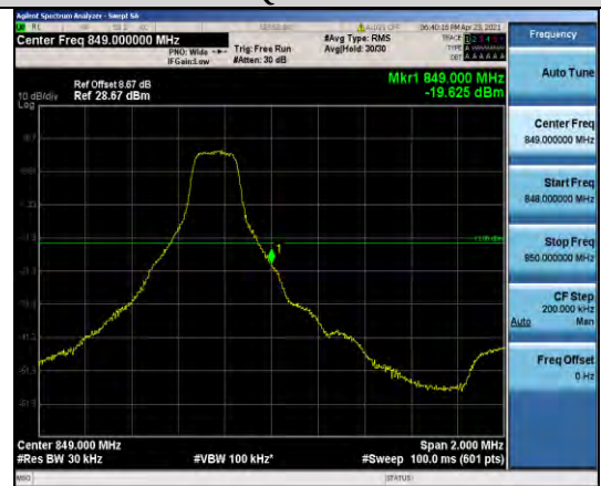
Band5-3MHz-QPSK-20635-1RB#14
