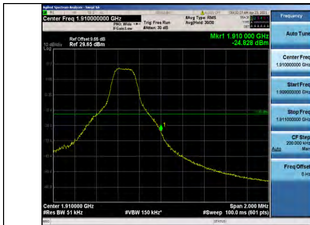
Band2-5MHz-QPSK-19175-1RB#24
