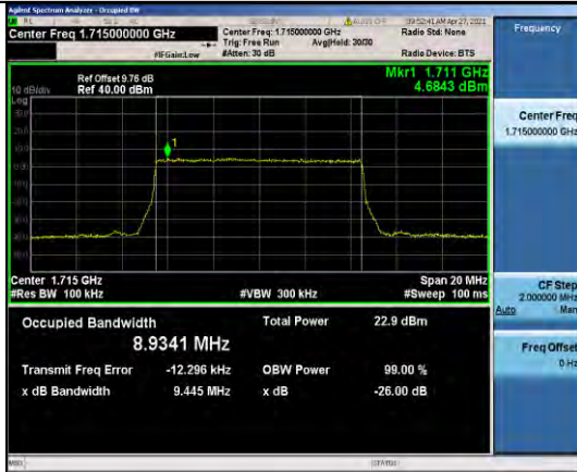
Band66-10MHz-QPSK-132022-50RB#0-8.9341
