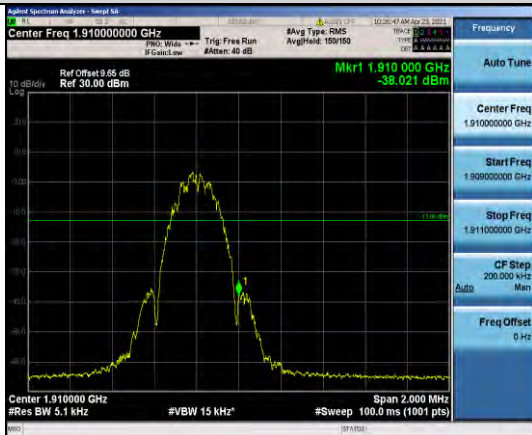
EGPRS1900-810
