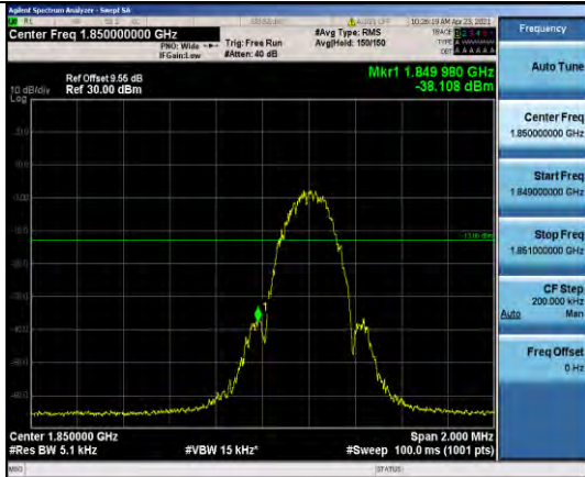
EGPRS1900-512
