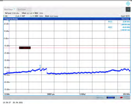
EGPRS1900-661-1000~20000MHz
