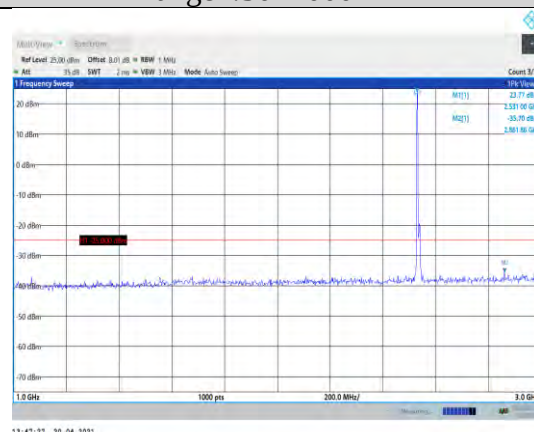
Band7-10MHz-QPSK-21100-1RB#0- Range2:1000~3000MHz
