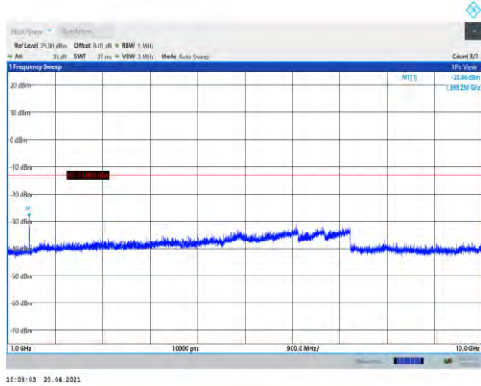
Band12-1.4MHz-QPSK-23017-1RB#0- Range2:1000~10000MHz
