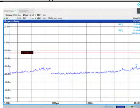
Band4-10MHz-QPSK-20350-1RB#0- Range2:1000~20000MHz
