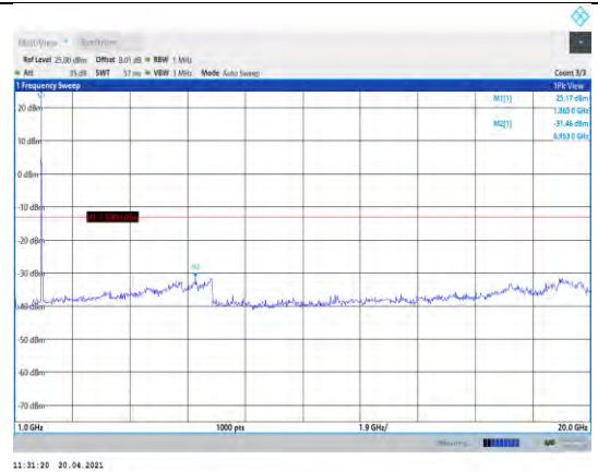
Band2-20MHz-QPSK-18900-1RB#0- Range2:1000~20000MHz
