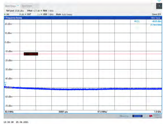
EGPRS1900-810-30~1000MHz
