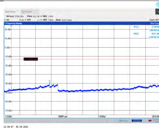
GSM1900-661-1000~20000MHz
