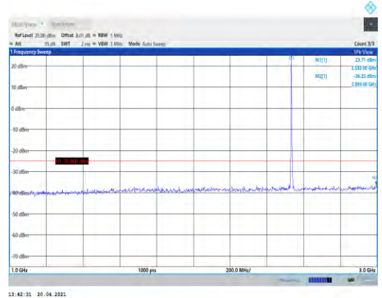
Band7-5MHz-QPSK-21100-1RB#0- Range2:1000~3000MHz
