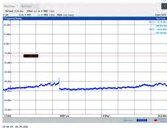
GSM1900-512-1000~20000MHz
