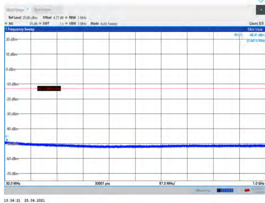
GSM1900-661-30~1000MHz
