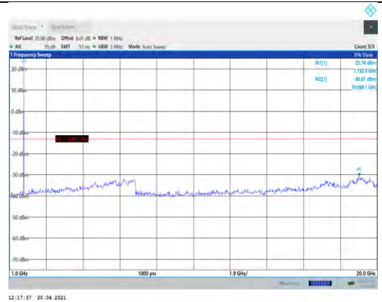
Band4-1.4MHz-QPSK-20175-1RB#0- Range2:1000~20000MHz
