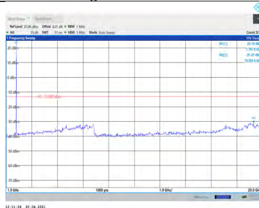
Band4-3MHz-QPSK-20385-1RB#0- Range2:1000~20000MHz
