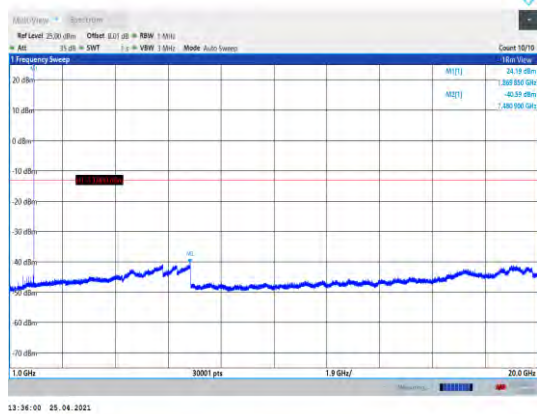
EGPRS1900-512-1000~20000MHz
