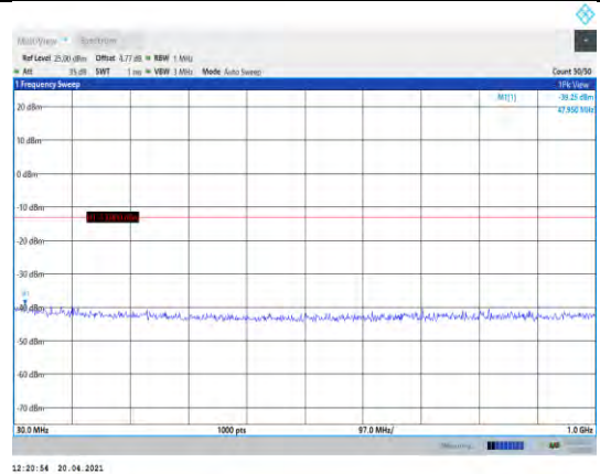
Band4-20MHz-QPSK-20300-1RB#0- Range1:30~1000MHz
