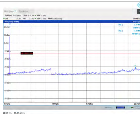
Band2-10MHz-QPSK-18900-1RB#0-Range2:1000~20000MHz
