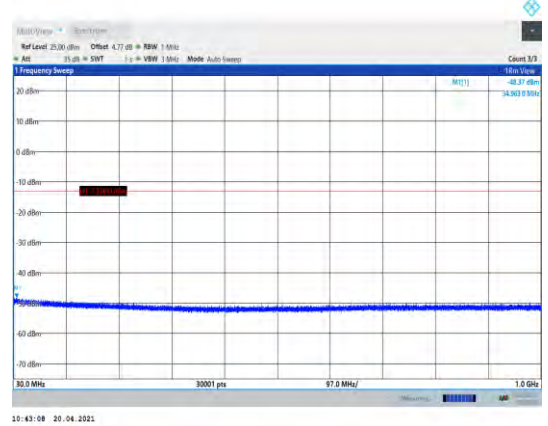
Band4-1513-30~1000MHz
