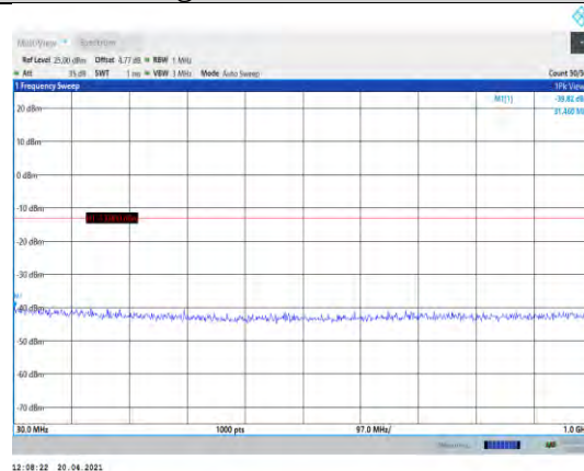
Band4-5MHz-QPSK-20375-1RB#0- Range1:30~1000MHz
