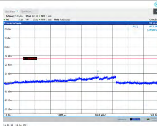
Band5-5MHz-QPSK-20525-1RB#0- Range2:1000~10000MHz
