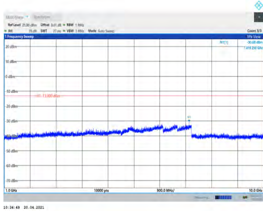
Band5-3MHz-QPSK-20415-1RB#0- Range2:1000~10000MHz
