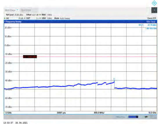
EGPRS850-251-1000~10000MHz
