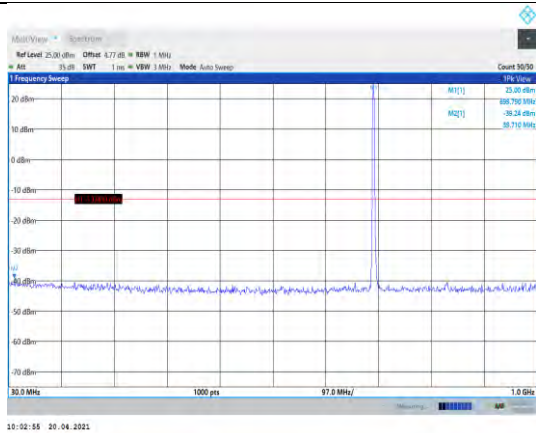
Band12-1.4MHz-QPSK-23017-1RB#0- Range1:30~1000MHz
