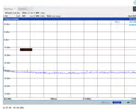
Band2-5MHz-QPSK-19175-1RB#0- Range1:30~1000MHz
