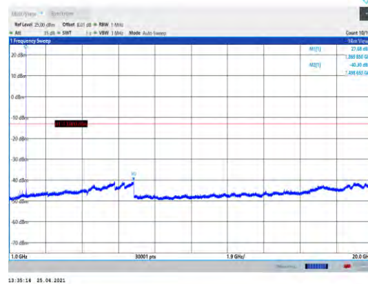
GSM1900-810-1000~20000MHz
