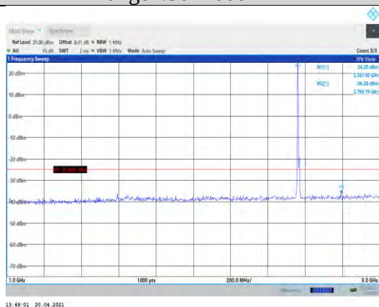
Band7-10MHz-QPSK-21400-1RB#0- Range2:1000~3000MHz
