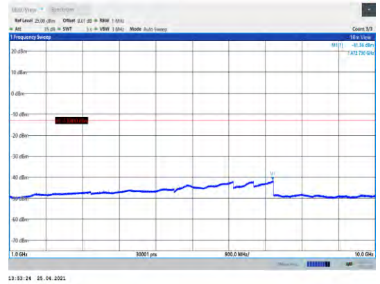
EGPRS850-190-1000~10000MHz
