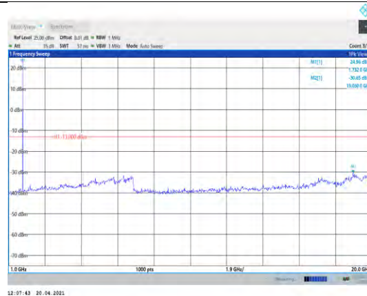
Band4-5MHz-QPSK-20175-1RB#0- Range2:1000~20000MHz
