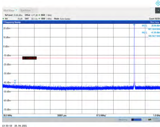
EGPRS850-190-30~1000MHz
