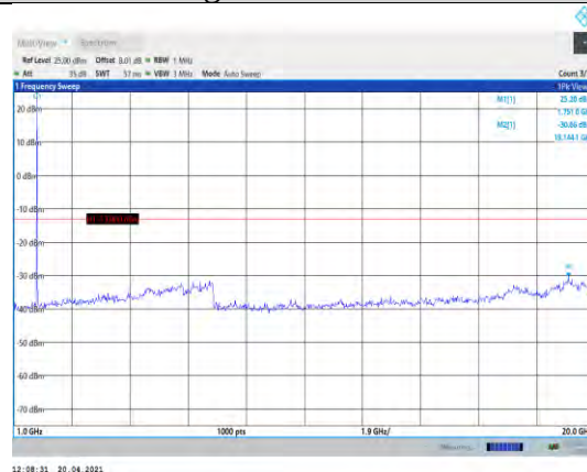
Band4-5MHz-QPSK-20375-1RB#0- Range2:1000~20000MHz
