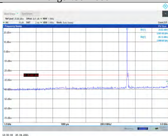
Band7-15MHz-QPSK-20825-1RB#0- Range2:1000~3000MHz
