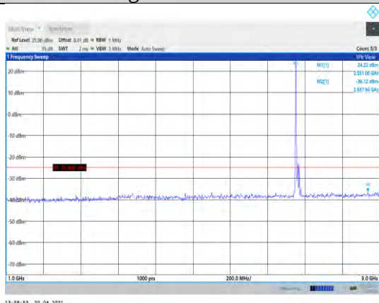
Band7-20MHz-QPSK-21350-1RB#0-Range2:1000~3000MHz
