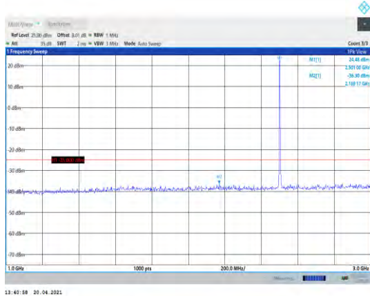
Band7-5MHz-QPSK-20775-1RB#0- Range2:1000~3000MHz
