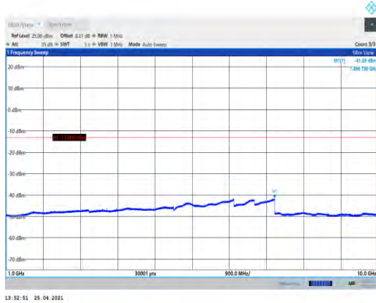
EGPRS850-128-1000~10000MHz
