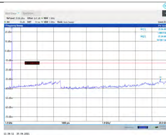
Band2-3MHz-QPSK-18900-1RB#0- Range2:1000~20000MHz
