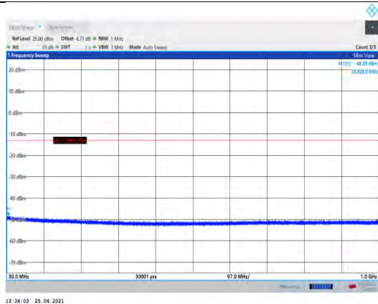
GSM1900-512-30~1000MHz
