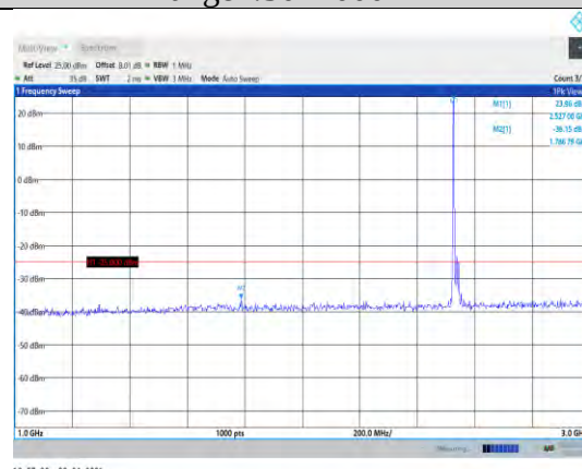
Band7-20MHz-QPSK-21100-1RB#0-Range2:1000~3000MHz
