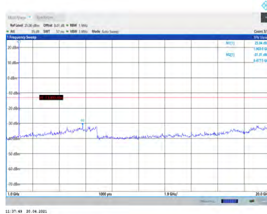
Band2-5MHz-QPSK-19175-1RB#0- Range2:1000~20000MHz
