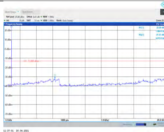
Band2-5MHz-QPSK-18900-1RB#0- Range2:1000~20000MHz
