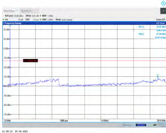
Band2-5MHz-QPSK-18625-1RB#0- Range2:1000~20000MHz
