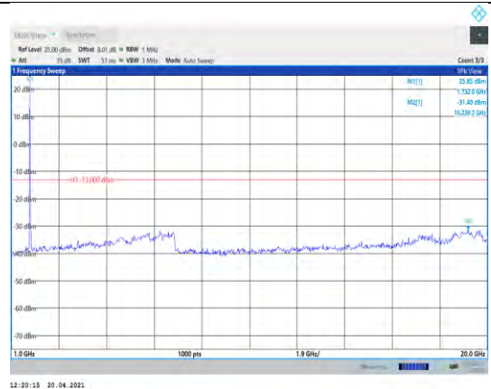
Band4-20MHz-QPSK-20175-1RB#0- Range2:1000~20000MHz
