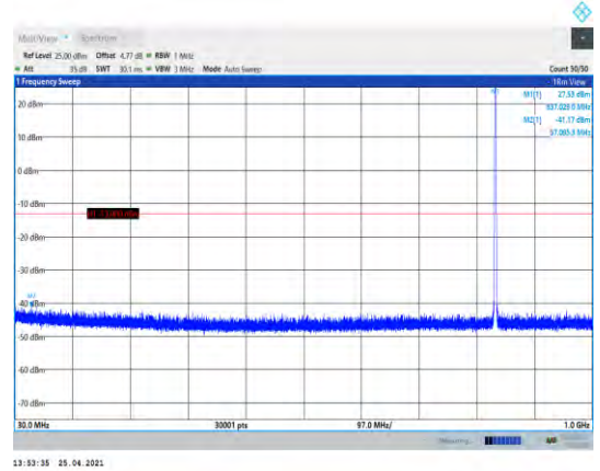
EGPRS850-251-30~1000MHz
