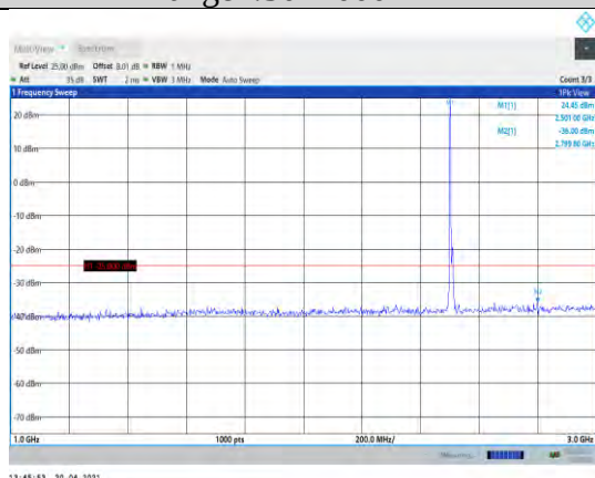
Band7-10MHz-QPSK-20800-1RB#0- Range2:1000~3000MHz
