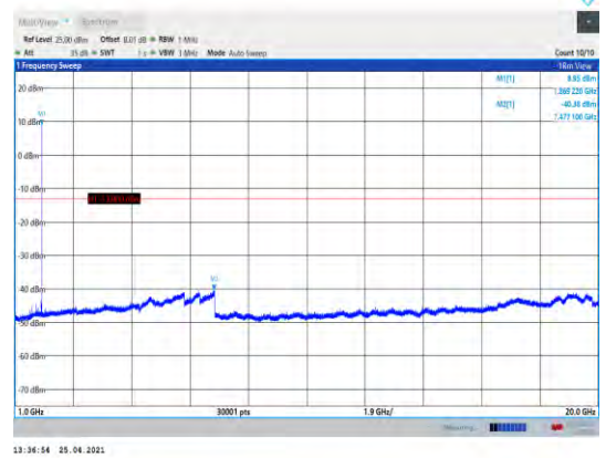
EGPRS1900-810-1000~20000MHz
