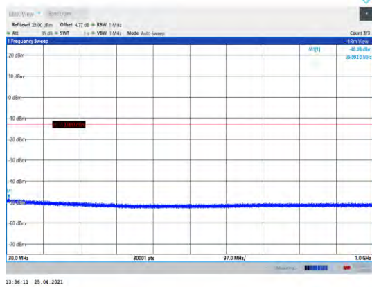
EGPRS1900-661-30~1000MHz
