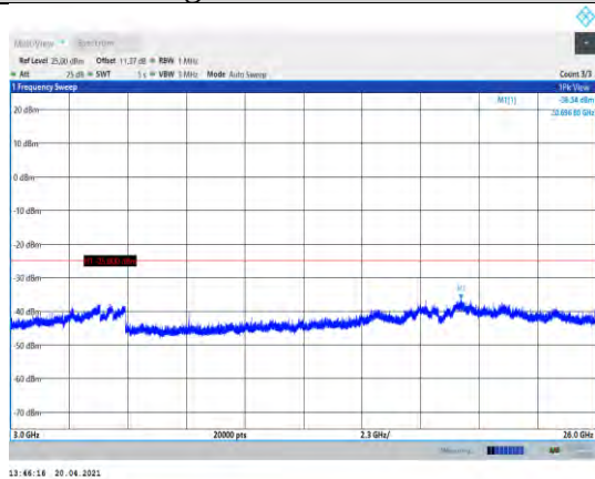
Band7-10MHz-QPSK-20800-1RB#0- Range3:3000~26000MHz
