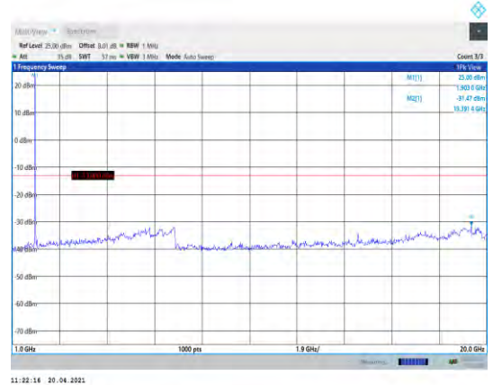
Band2-15MHz-QPSK-19125-1RB#0- Range2:1000~20000MHz
