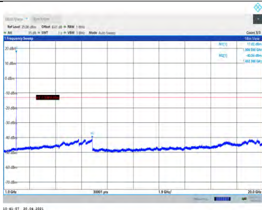
Band2-9538-1000~20000MHz
