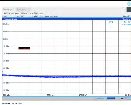
EGPRS1900-512-30~1000MHz
