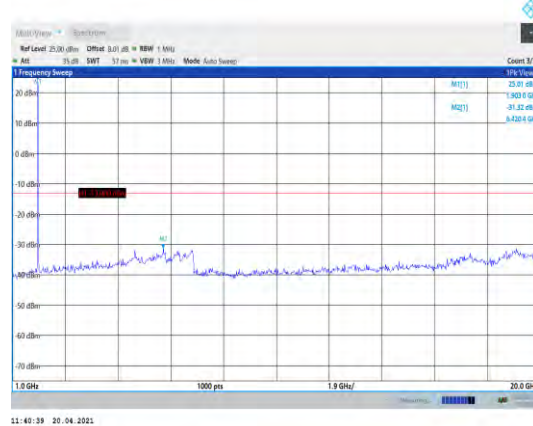
Band2-10MHz-QPSK-19150-1RB#0-Range2:1000~20000MHz
