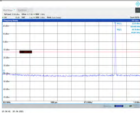
Band5-3MHz-QPSK-20415-1RB#0- Range1:30~1000MHz
