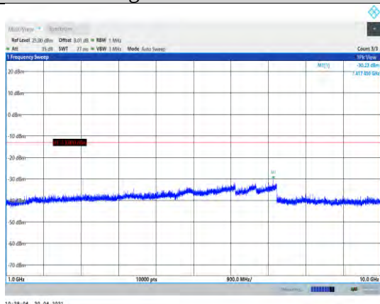
Band5-5MHz-QPSK-20425-1RB#0- Range2:1000~10000MHz
