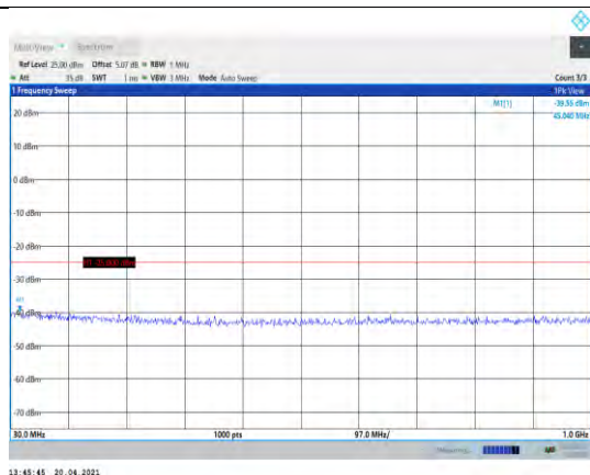
Band7-10MHz-QPSK-20800-1RB#0- Range1:30~1000MHz
