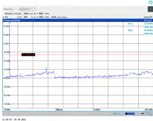
Band2-10MHz-QPSK-18650-1RB#0-Range2:1000~20000MHz
