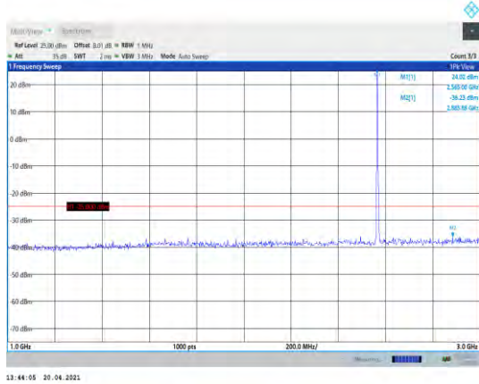
Band7-5MHz-QPSK-21425-1RB#0- Range2:1000~3000MHz
