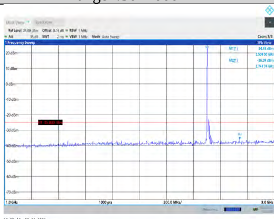
Band7-20MHz-QPSK-20850-1RB#0-Range2:1000~3000MHz
