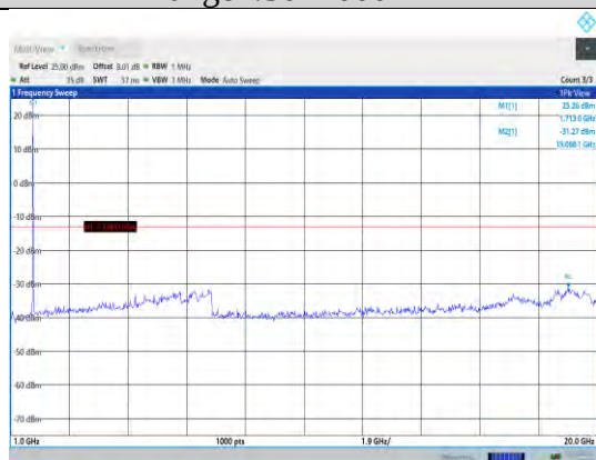
Band4-10MHz-QPSK-20000-1RB#0- Range2:1000~20000MHz
