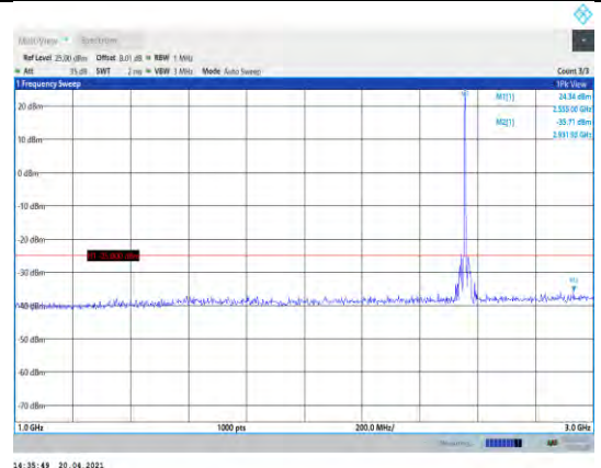
Band41-5MHz-QPSK-40265-1RB#0-Range2:1000~3000MHz
