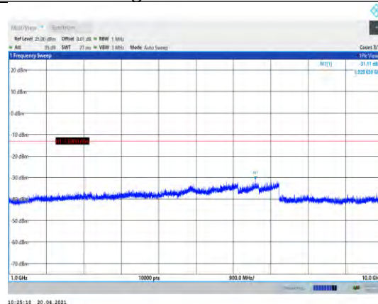
Band26-3MHz-QPSK-26775-1RB#0- Range2:1000~10000MHz
