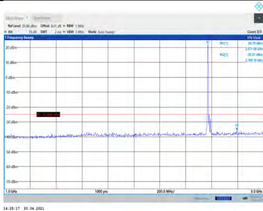
Band38-20MHz-16QAM-37850-1RB#0- Range2:1000~3000MHz
