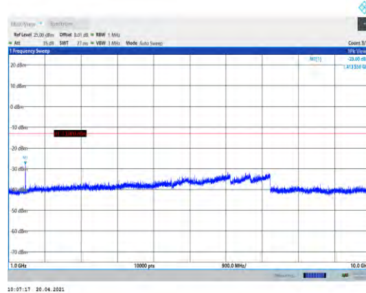
Band12-10MHz-QPSK-23130-1RB#0- Range2:1000~10000MHz
