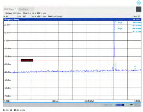
Band38-5MHz-QPSK-38225-1RB#0-Range2:1000~3000MHz
