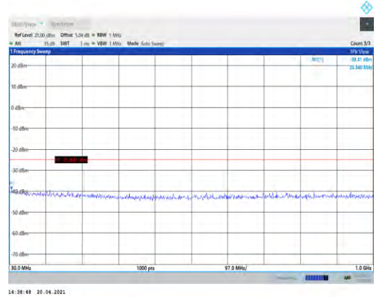
Band41-5MHz-QPSK-41215-1RB#0- Range1:30~1000MHz
