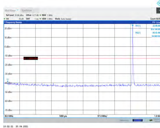
Band26-5MHz-QPSK-26765-1RB#0- Range1:30~1000MHz
