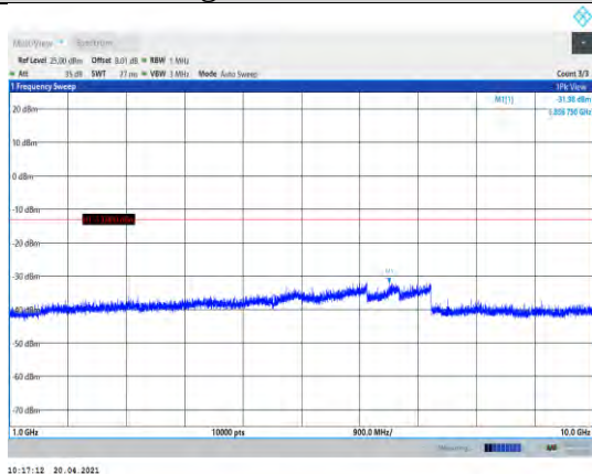
Band26-1.4MHz-QPSK-26697-1RB#0-Range2:1000~10000MHz
