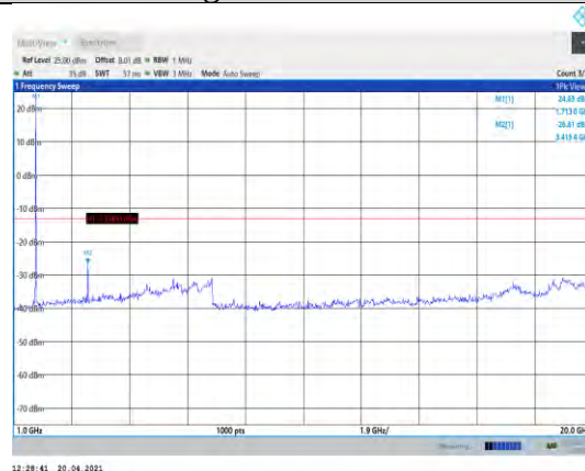
Band66-5MHz-QPSK-131997-1RB#0-Range2:1000~20000MHz
