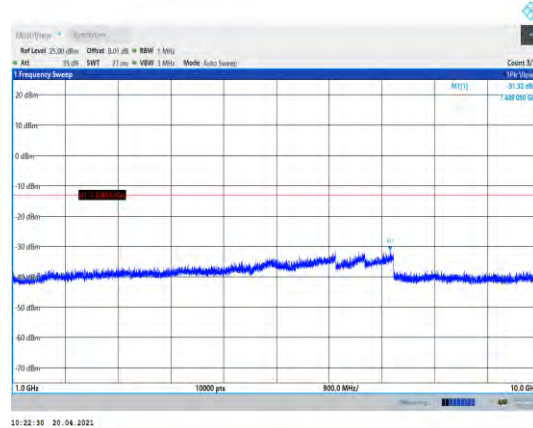
Band26-5MHz-QPSK-26765-1RB#0- Range2:1000~10000MHz
