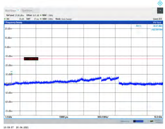
Band12-5MHz-QPSK-23155-1RB#0- Range2:1000~10000MHz
