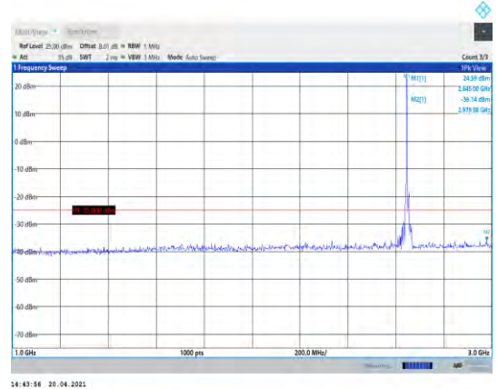
Band41-10MHz-QPSK-41190-1RB#0- Range2:1000~3000MHz
