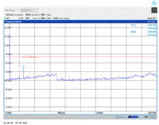
Band66-3MHz-QPSK-131987-1RB#0- Range2:1000~20000MHz
