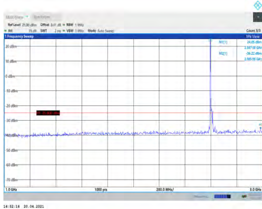
Band41-20MHz-QPSK-40740-1RB#0-Range2:1000~3000MHz
