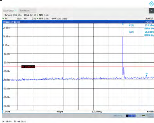
Band38-20MHz-QPSK-38000-1RB#0- Range2:1000~3000MHz
