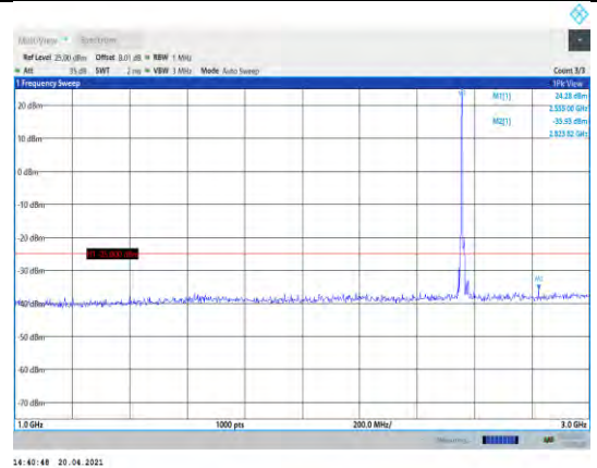
Band41-10MHz-QPSK-40290-1RB#0- Range2:1000~3000MHz
