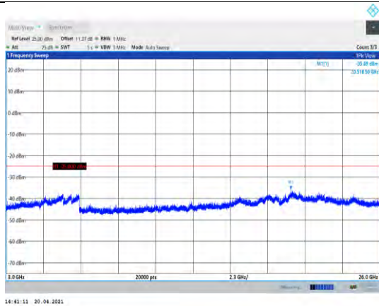
Band41-10MHz-QPSK-40290-1RB#0- Range3:3000~26000MHz
