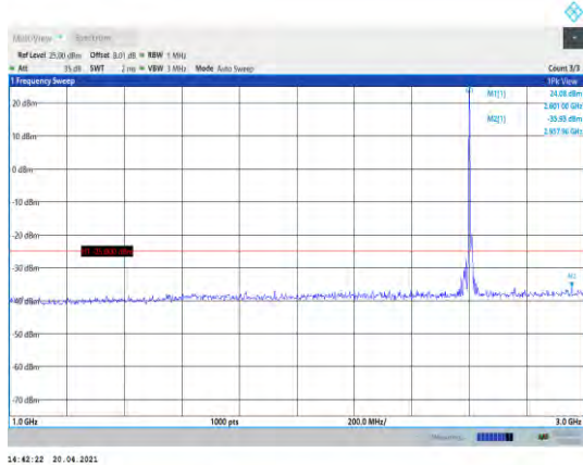
Band41-10MHz-QPSK-40740-1RB#0- Range2:1000~3000MHz
