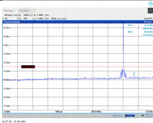
Band41-5MHz-QPSK-40740-1RB#0- Range2:1000~3000MHz
