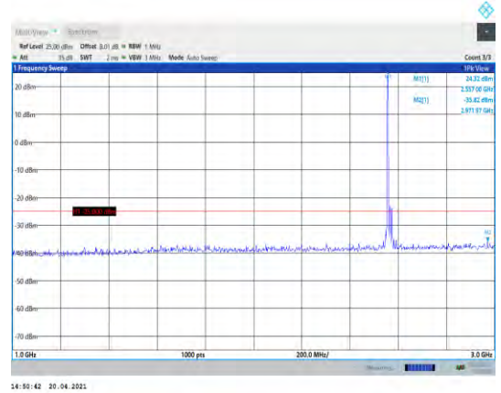
Band41-20MHz-QPSK-40340-1RB#0- Range2:1000~3000MHz
