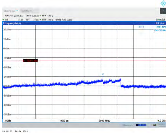
Band26-5MHz-QPSK-26715-1RB#0- Range2:1000~10000MHz
