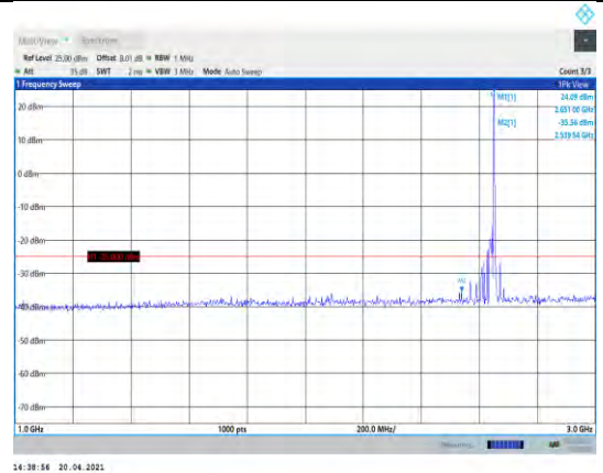
Band41-5MHz-QPSK-41215-1RB#0- Range2:1000~3000MHz
