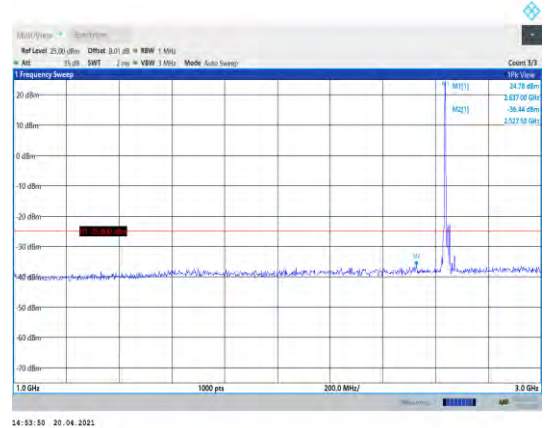
Band41-20MHz-QPSK-41140-1RB#0-Range2:1000~3000MHz
