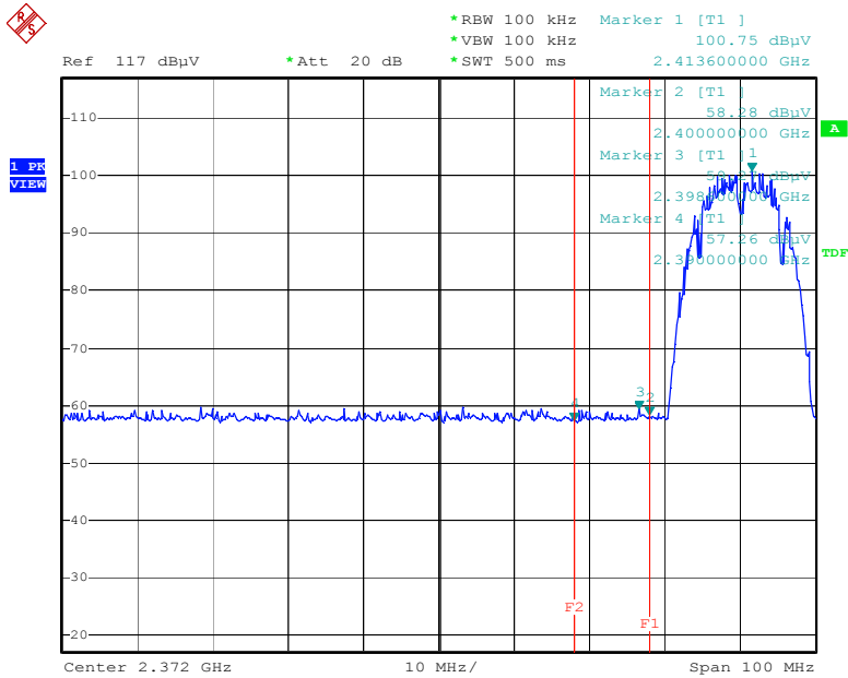
IEEE 802.11b Channel: Low
