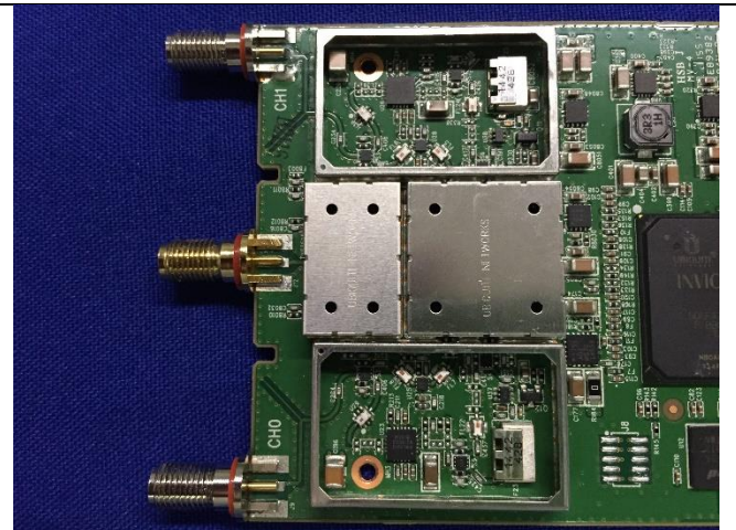
EUT - Radio Module View
