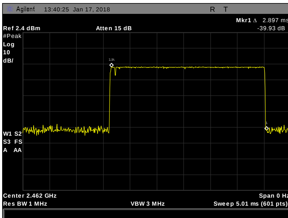
Plot 20. DH5 Pulse Width
