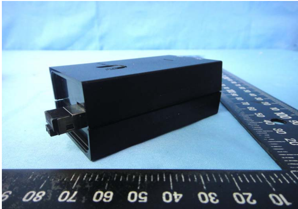
(6) EUT Photo
