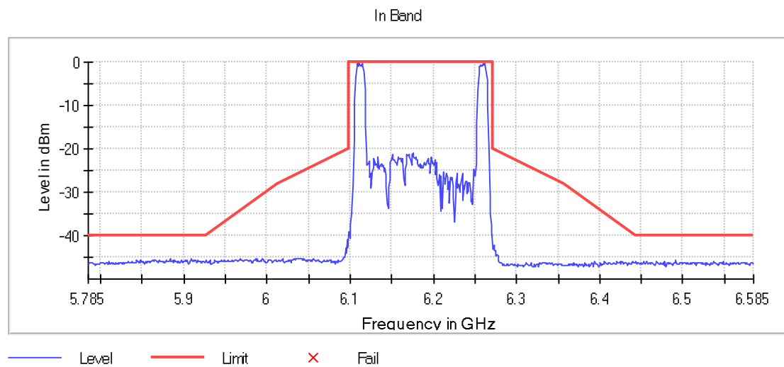
Figure 12: 6185 160MHz RU Vérification - Edge
