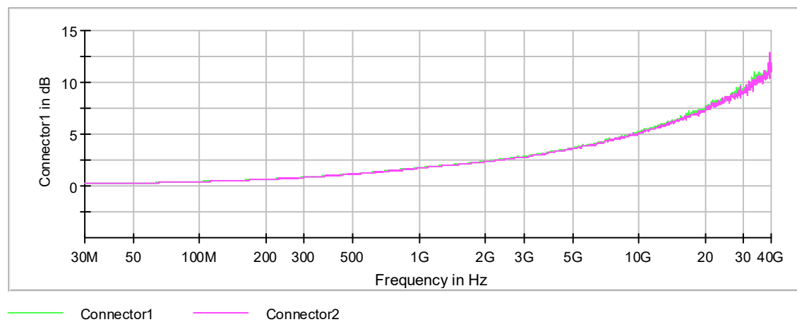
Attenuation
