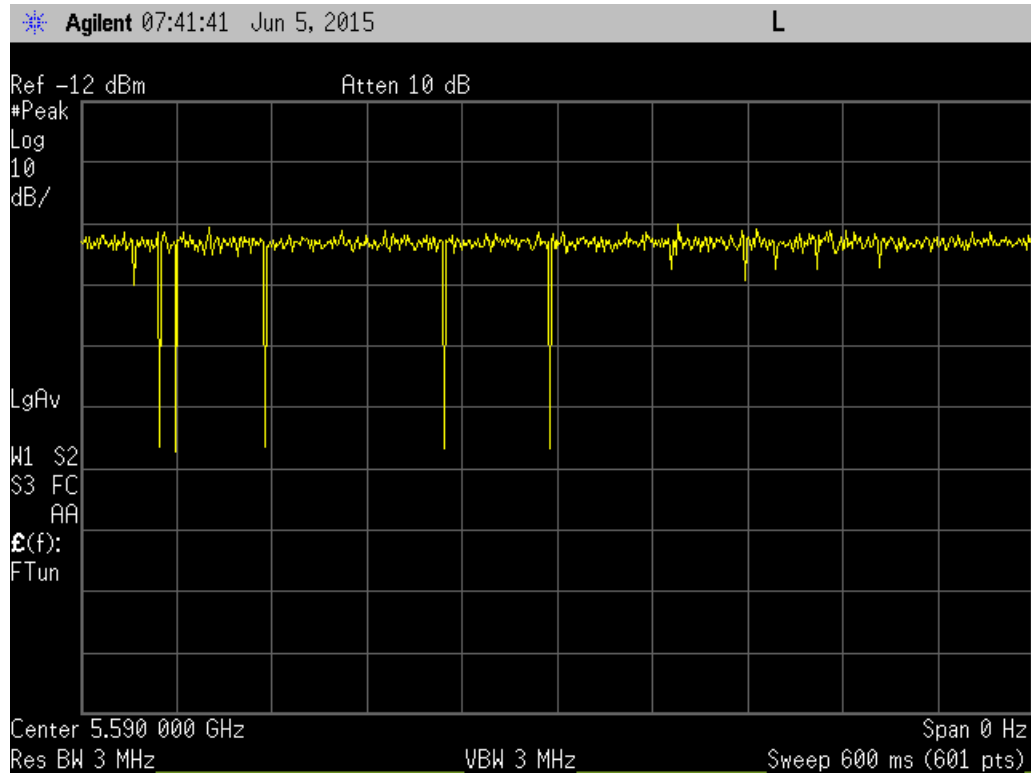
20MHz Bandwidth
