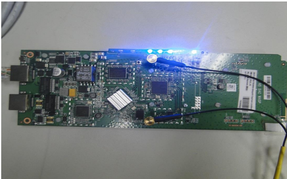
EUT
