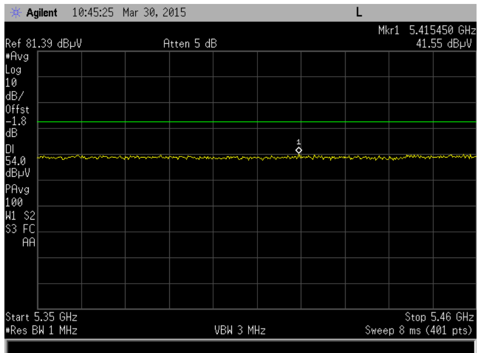
80MHz mid ch 5350-5460MHz J8
