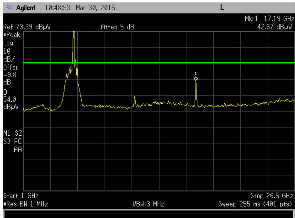
10MHz low ch 1-26.5GHz J8
