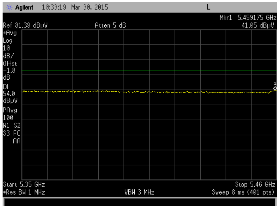
50MHz mid ch 5350-5460MHz J8
