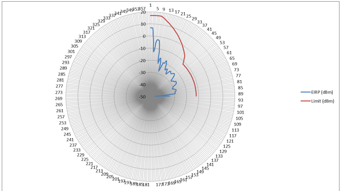
RD-5G30 – Horizontal
