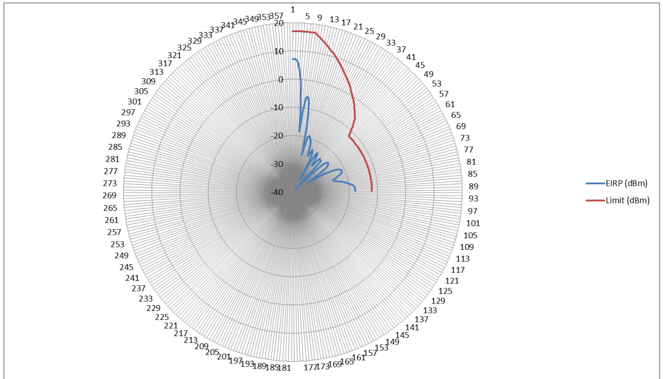
RD-5G30 – Horizontal
