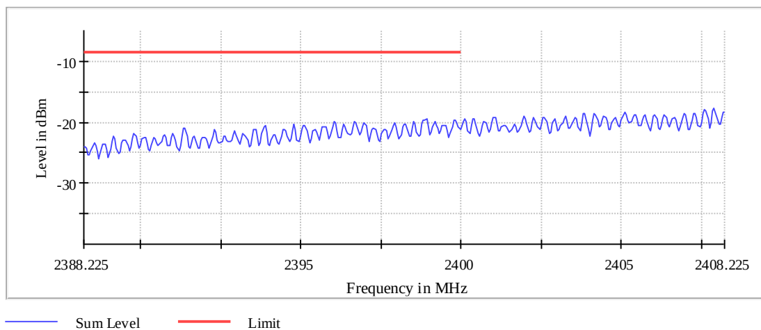
FinalMeas_2398225000Hz
