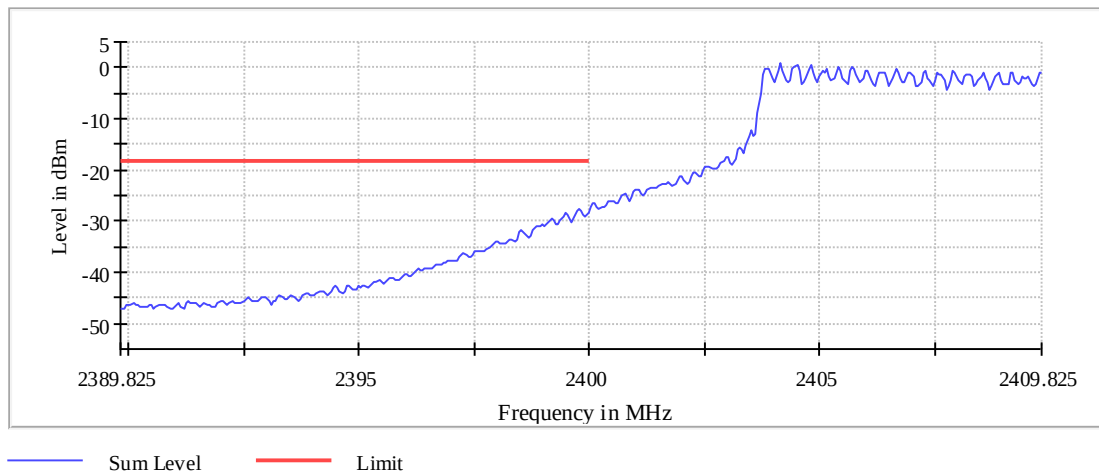
FinalMeas_2399825000Hz
