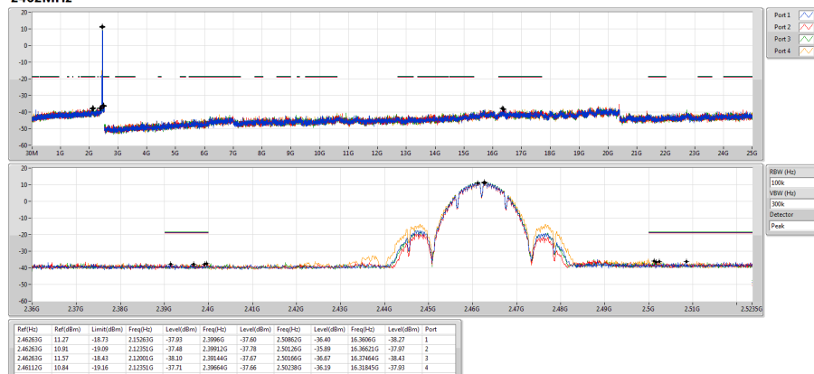
802.11b_Nss1,(1Mbps)_4TX 2462MHz
