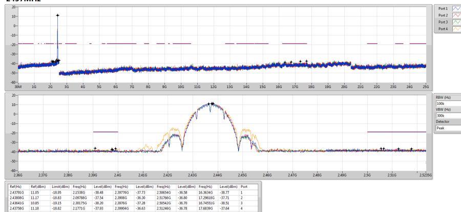
802.11b_Nss1,(1Mbps)_4TX 2437MHz
