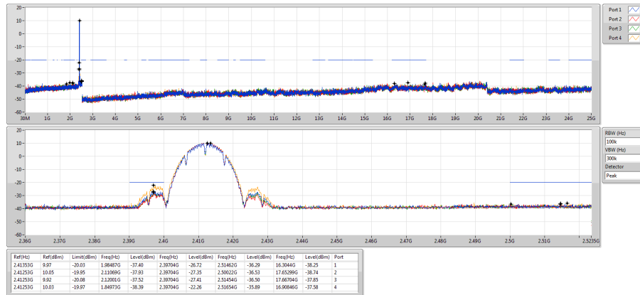
802.11b_Nss1,(1Mbps)_4TX 2412MHz
