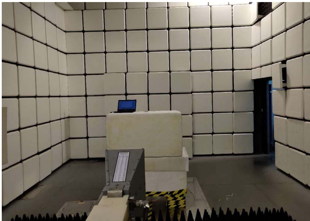
1GHz-18GHz
