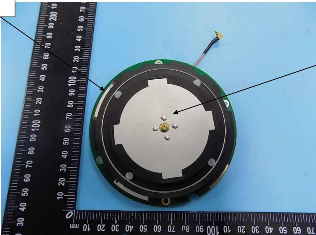
GPS Ant
