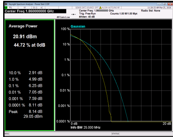
Band2 16QAM BW=20MHz Channel=18700 RB Size=100 Position=#0
