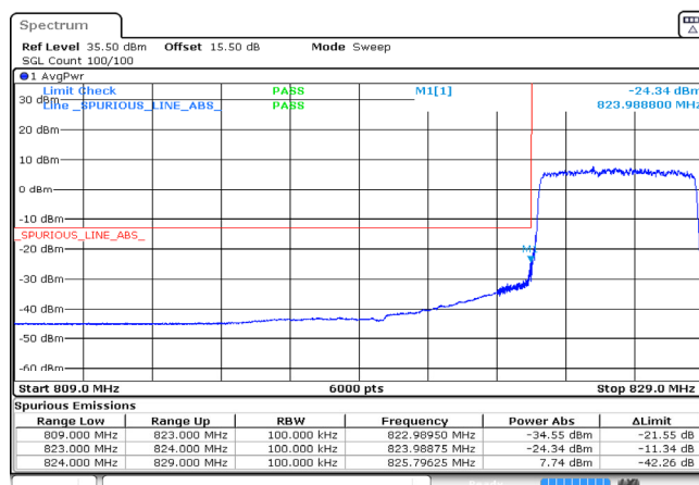
5MHz_Low_QPSK_25@0 -24.34dBm
