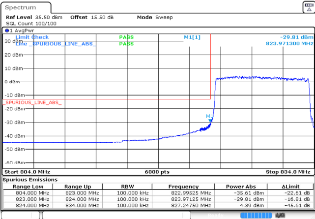
10MHz_Low_QPSK_50@0 -29.81dBm
