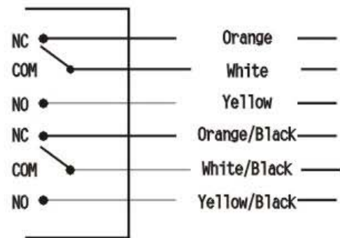
F1:Car Alarm Out-Port
