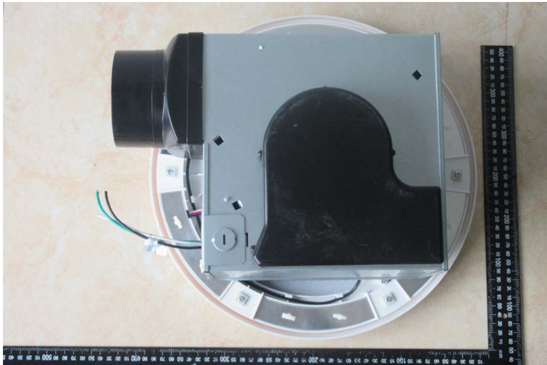
(6) Fan bottom view
