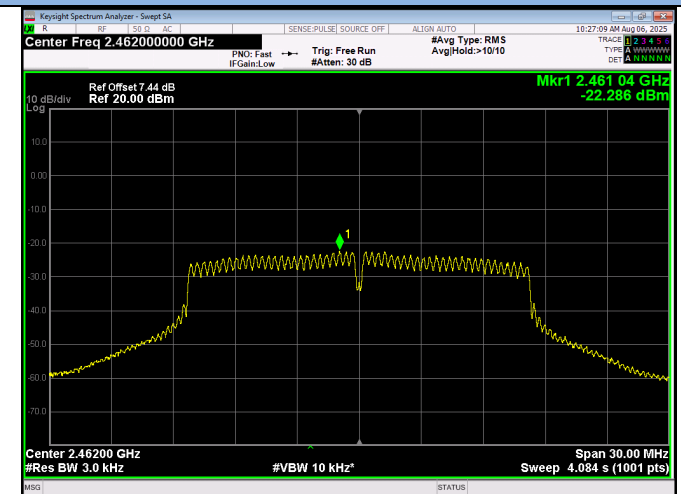
IEEE 802.11g - 2462MHz
