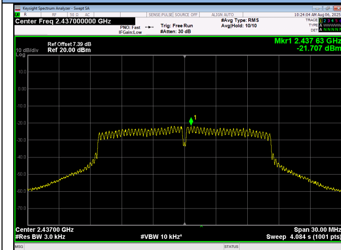
IEEE 802.11g - 2437MHz
