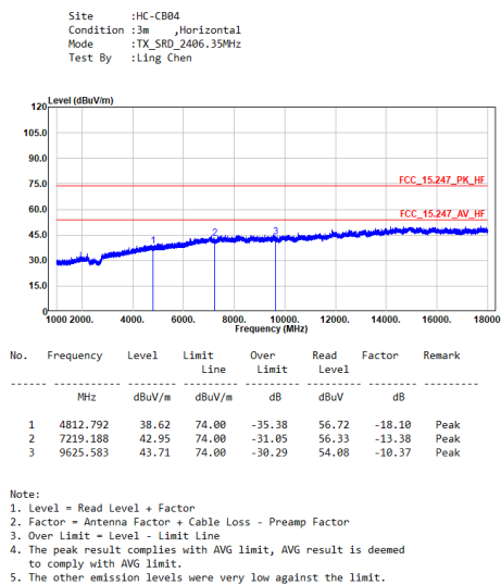
TX_SRD_2406.35MHz_H
