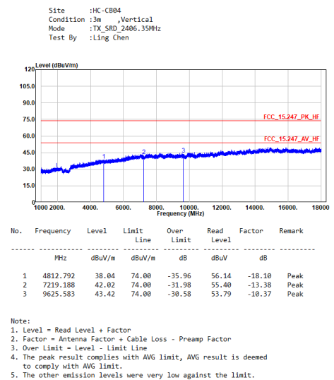
TX_SRD_2406.35MHz_V
