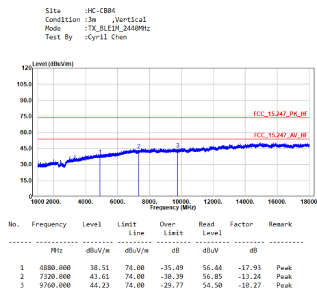
TX_BLE1M_2440MHz_V
