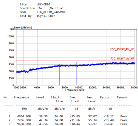
TX_BLE1M_2402MHz_V
