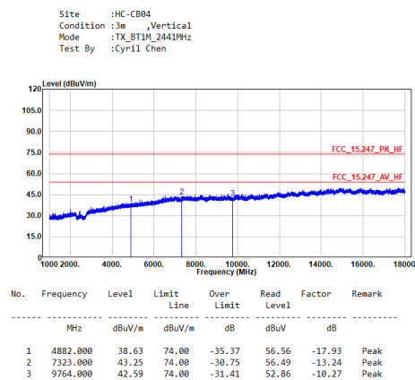
TX_BT1M_2441MHz_V
