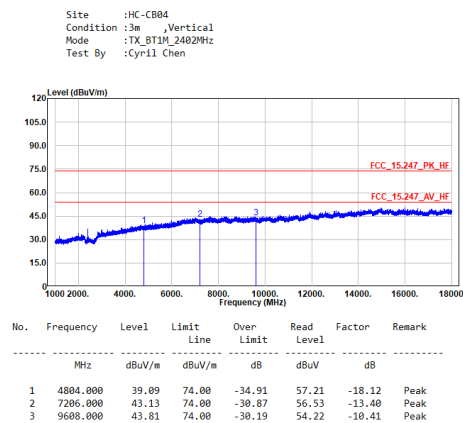
TX_BT1M_2402MHz_V
