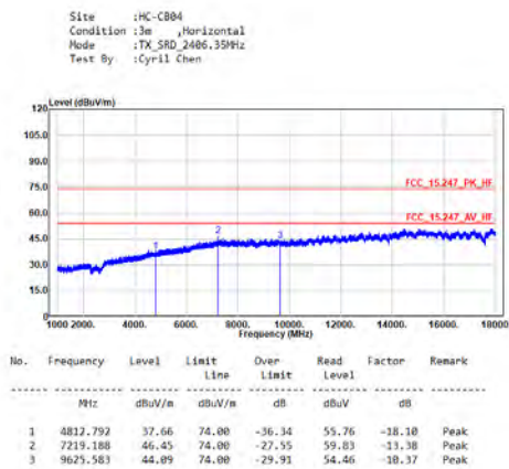
TX_SRD_2406.35MHz_H
