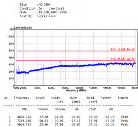
TX_SRD_2406.35MHz_V
