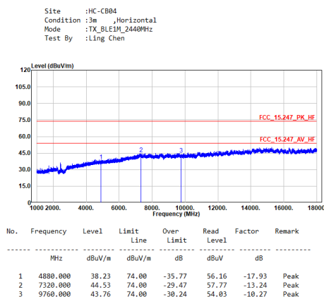
TX_BLE1M_2440MHz_H
