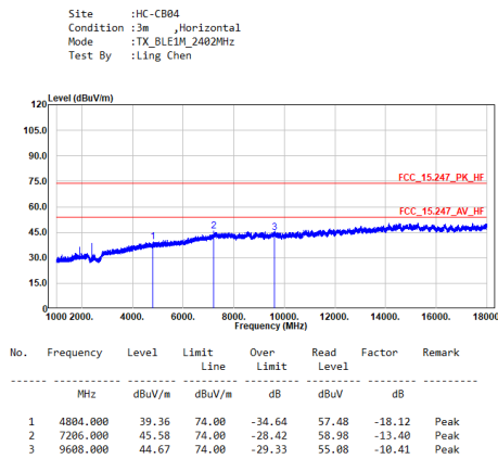
TX_BLE1M_2402MHz_H
