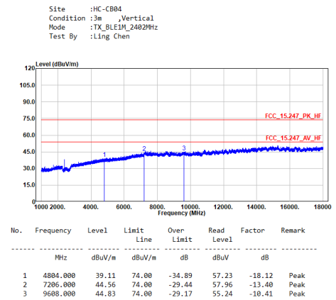
TX_BLE1M_2402MHz_V
