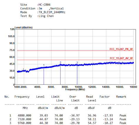
TX_BLE1M_2440MHz_V
