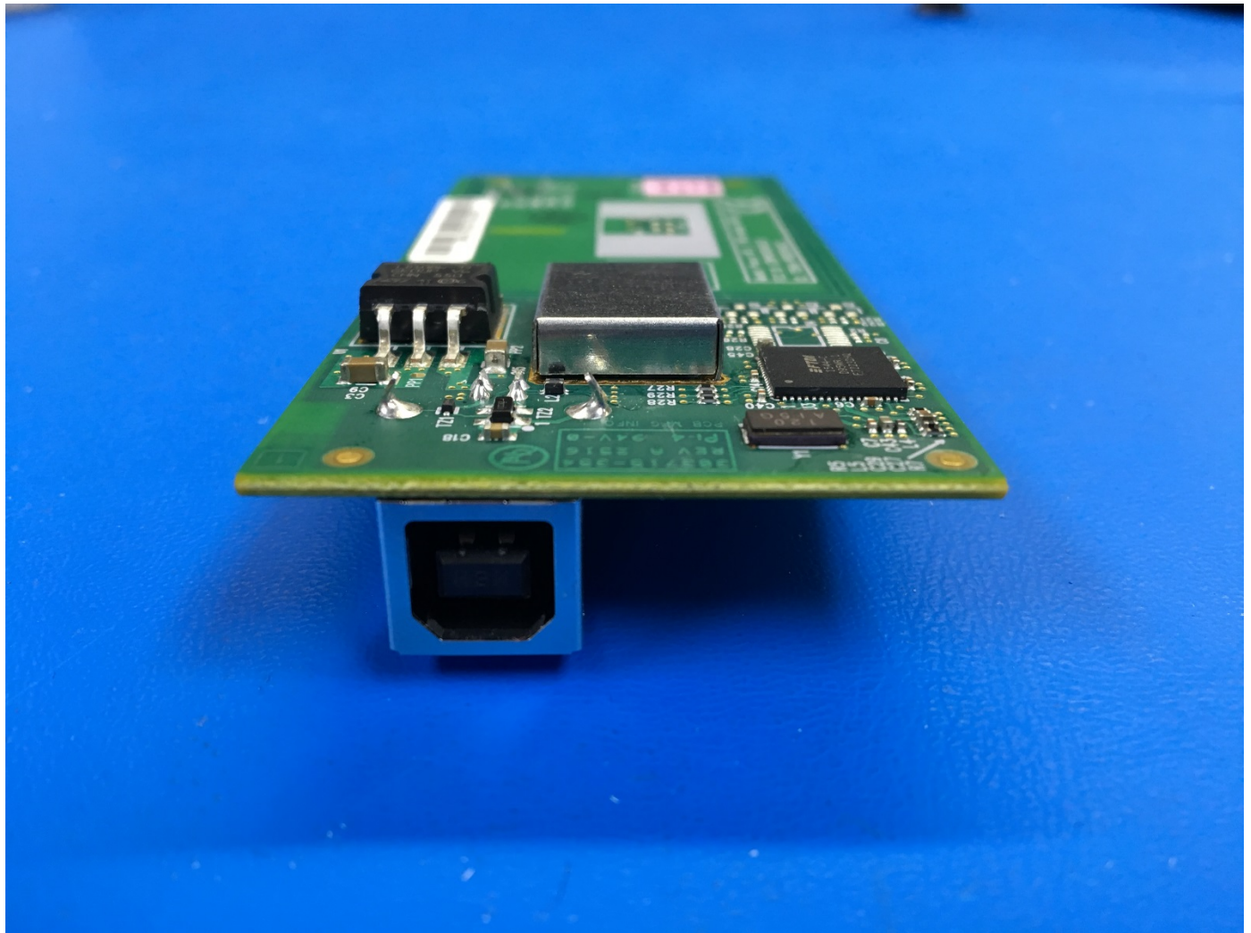
Precor NFC / RFID Module 304232 internal photos
