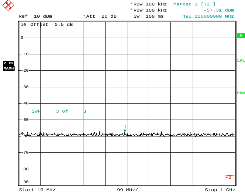
Plot No: 4.8
