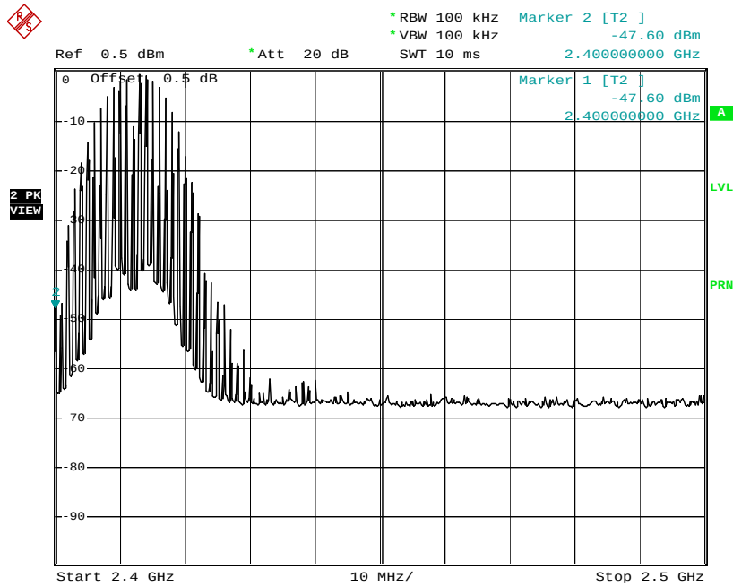
Plot No: 4.27
