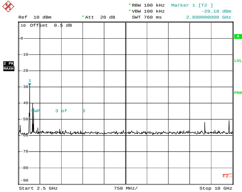
Plot No: 4.11
