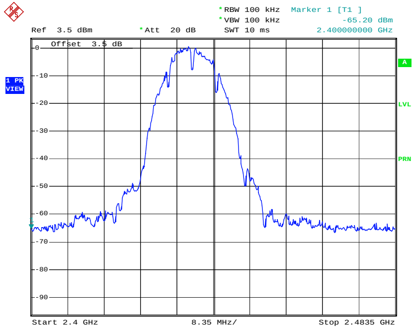
Plot No: 4.13
