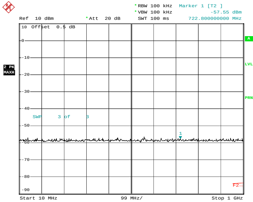
Plot No: 4.15
