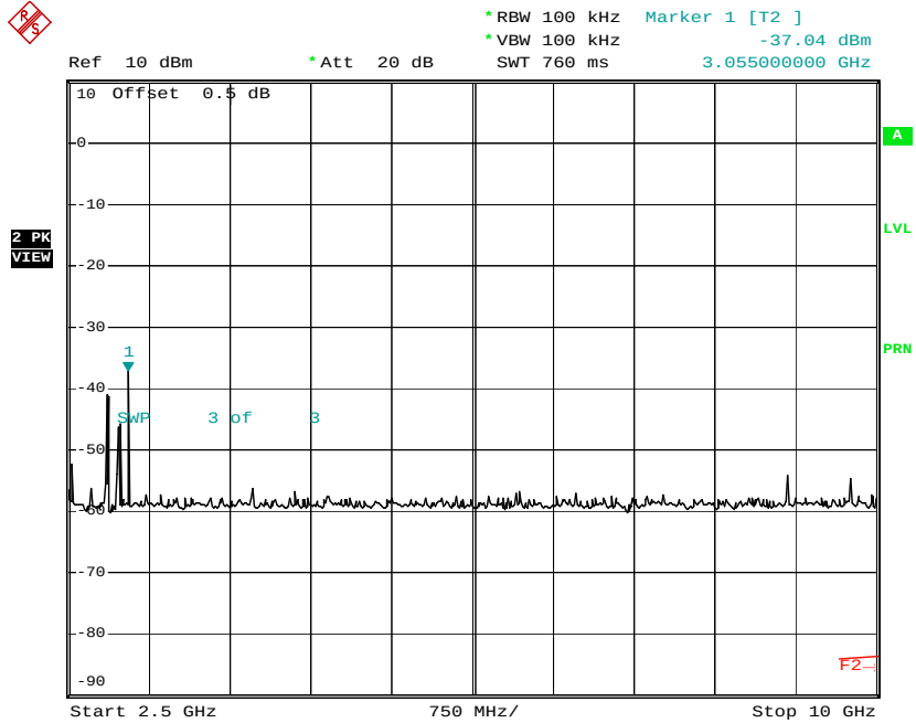
Plot No: 4.4
