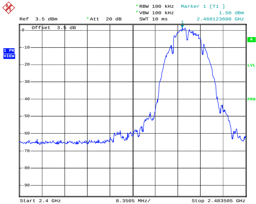
Plot No: 4.20
