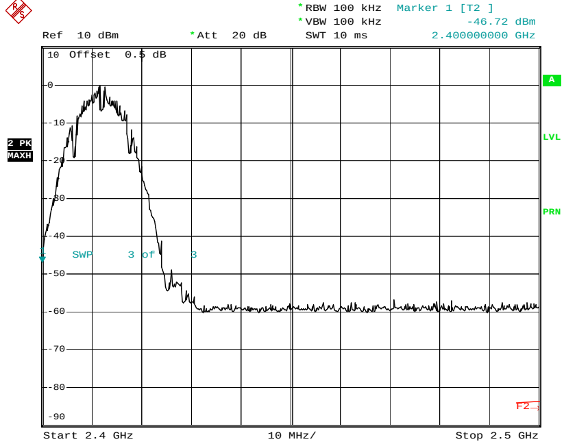
Plot No: 4.7
