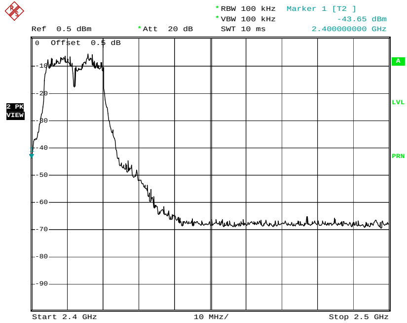
Plot No: 4.24
