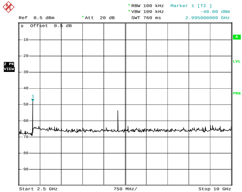
Plot No: 4.25
