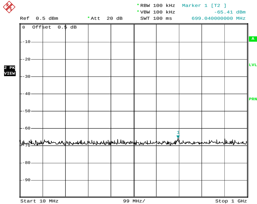
Plot No: 4.29
