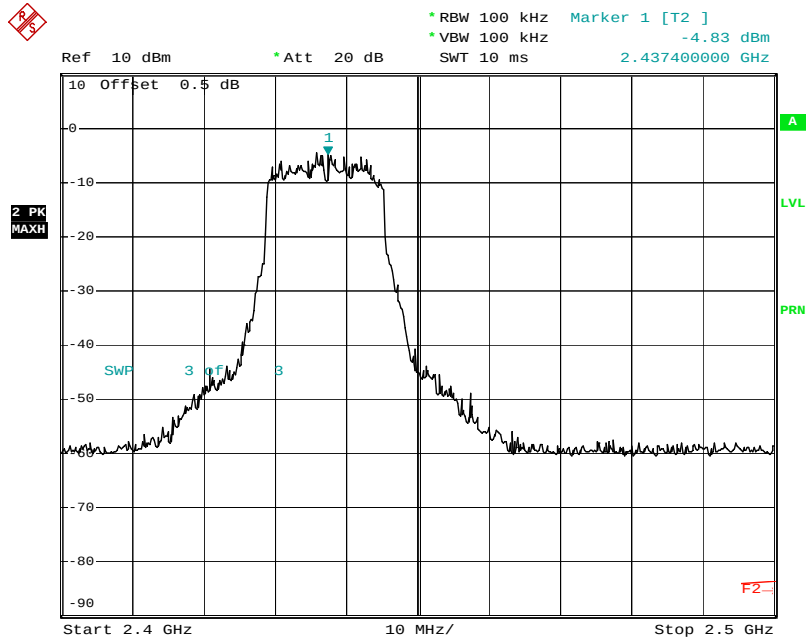
Plot No: 4.10
