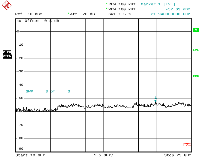
Plot No: 4.5
