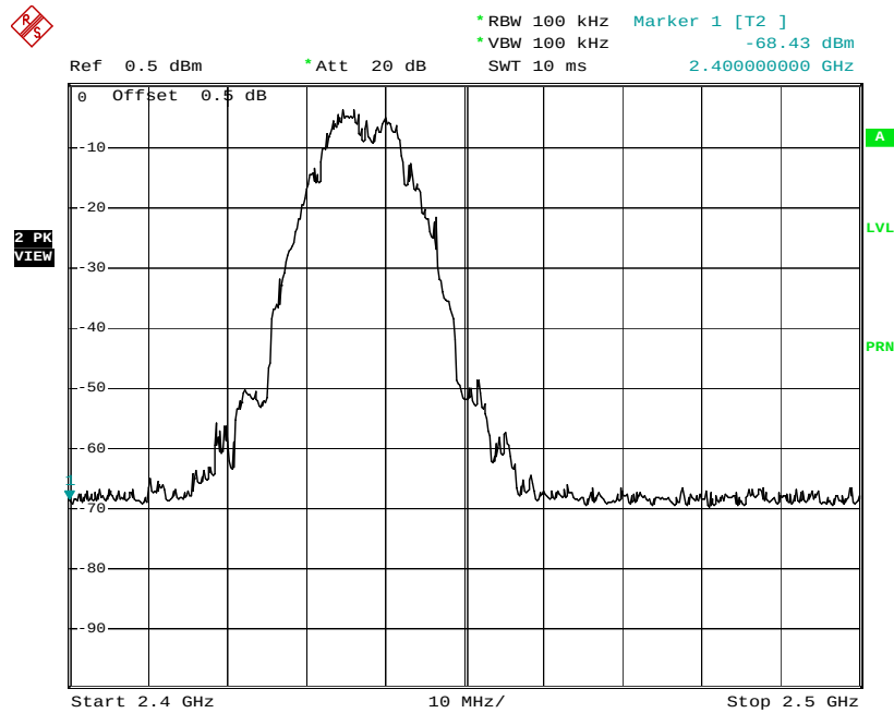
Plot No: 4.35
