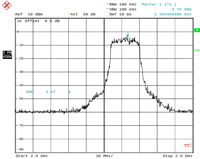
Plot No: 4.17
