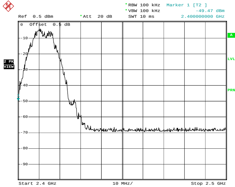
Plot No: 4.28
