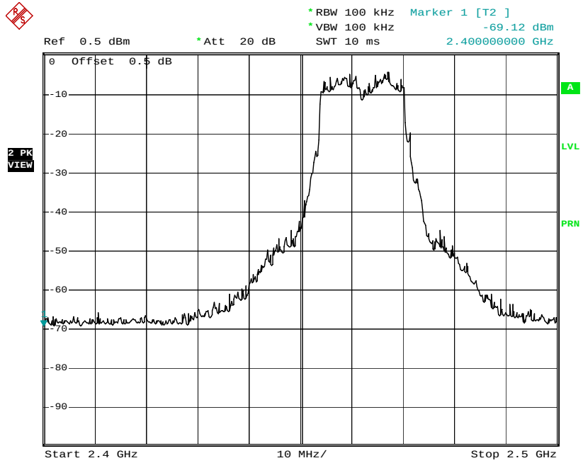
Plot No: 4.38
