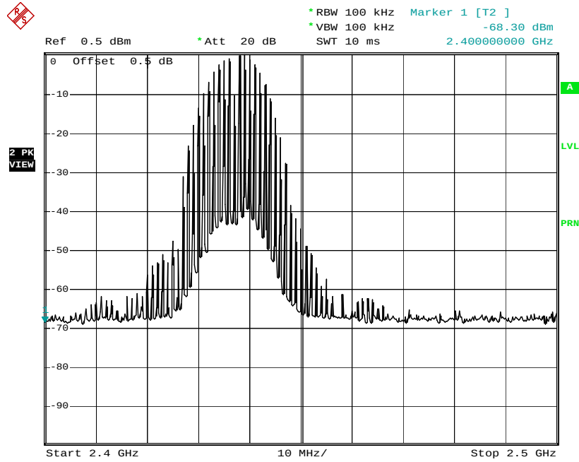
Plot No: 4.34
