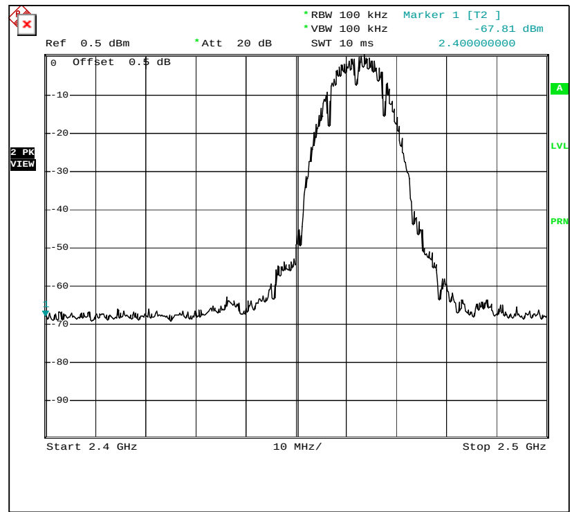
Plot No: 4.41
