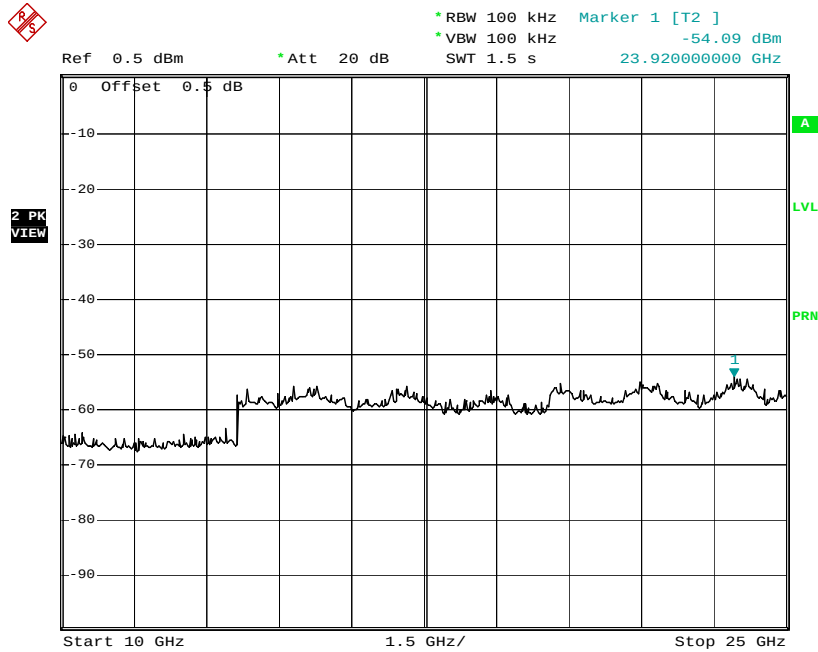
Plot No: 4.26
