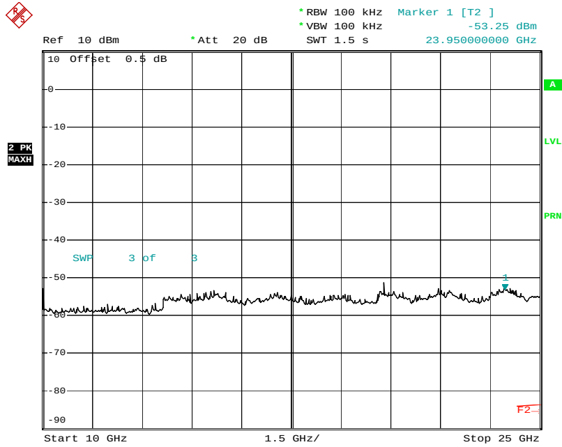
Plot No: 4.19
