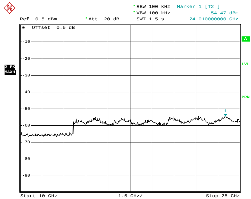
Plot No: 4.40
