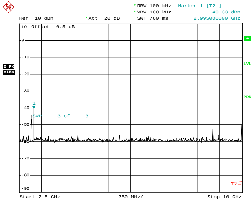
Plot No: 4.18
