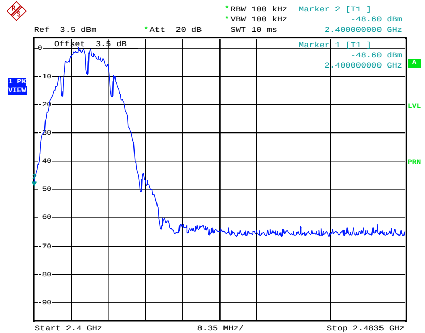
Plot No: 4.6
