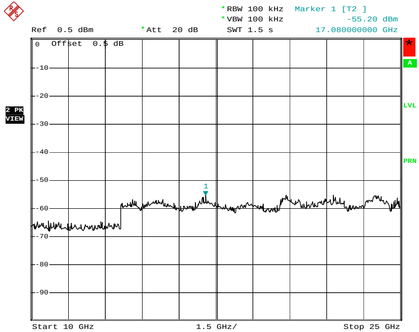
Plot No: 4.33
