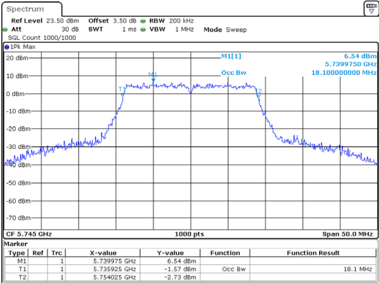
802.11ac20_5745MHz
