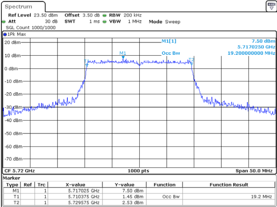
802.11ax20_5720MHz_RU_Full
