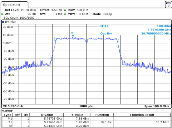
802.11ac40_5795MHz
