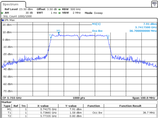
802.11ac40_5755MHz
