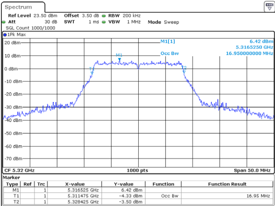
802.11a_5320MHz
