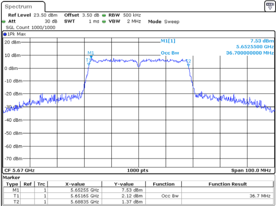
802.11ac40_5670MHz
