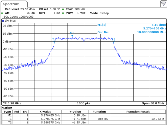
802.11ac20_5280MHz
