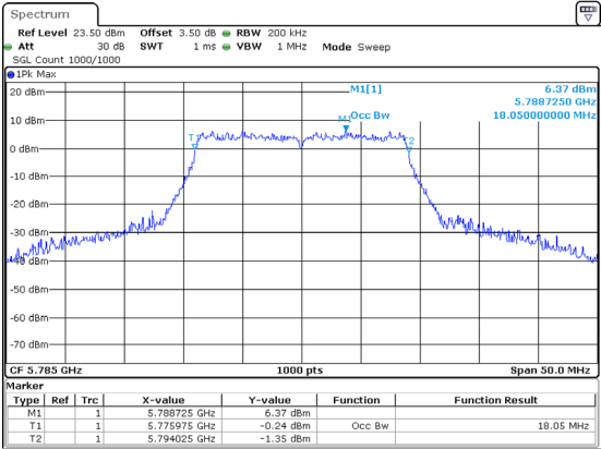
802.11ac20_5785MHz
