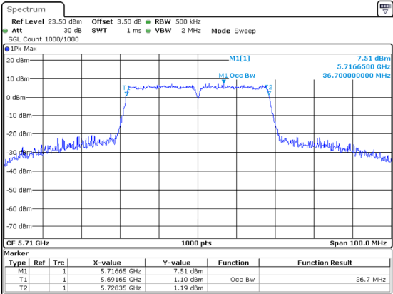
802.11ac40_5710MHz
