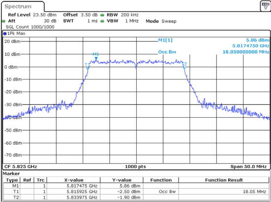
802.11ac20_5825MHz
