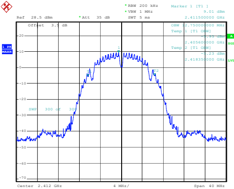
802.11b_2412MHz
