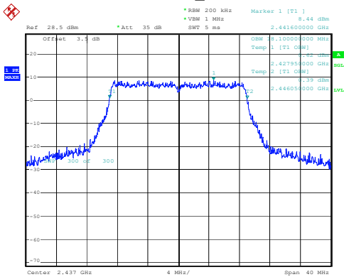
802.11n20_2437MHz
