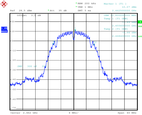
802.11b_2462MHz
