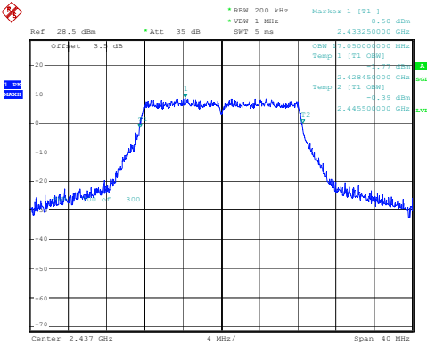
802.11g_2437MHz
